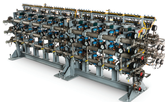
Сдвоенный манифольд с 9 входами и 5 выходами, используемый для перекачки продукта в секцию упаковки и распределения.
