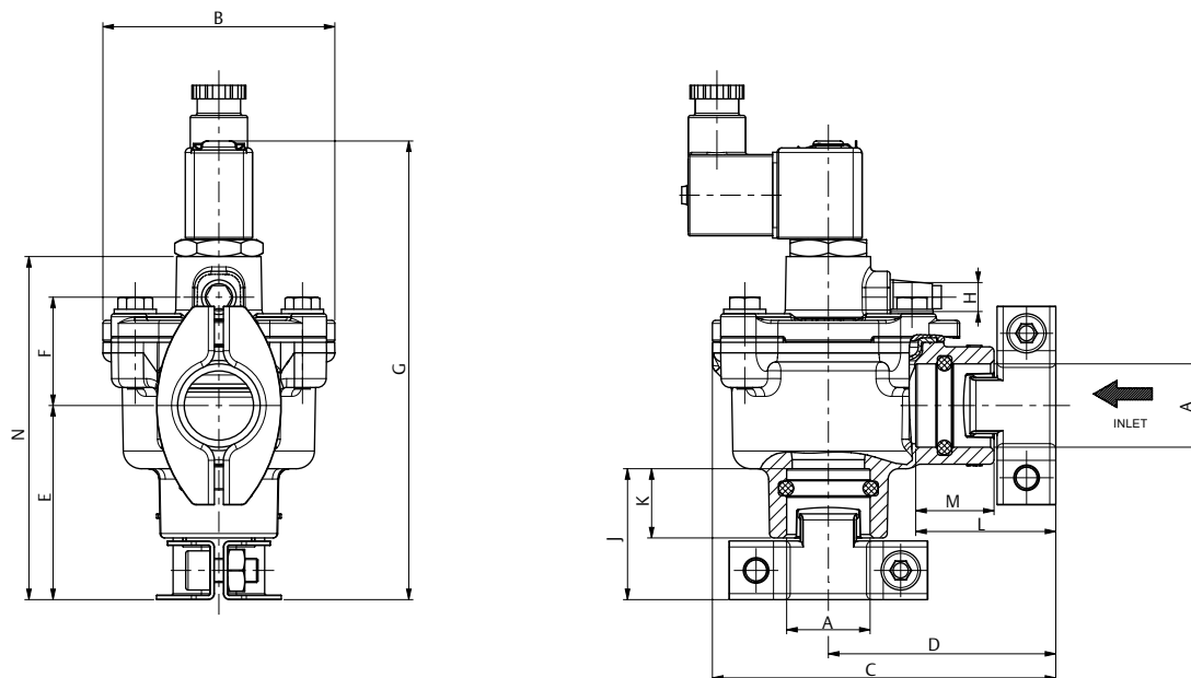
Рис. 2. Пневмоуправляемый импульсный клапан
