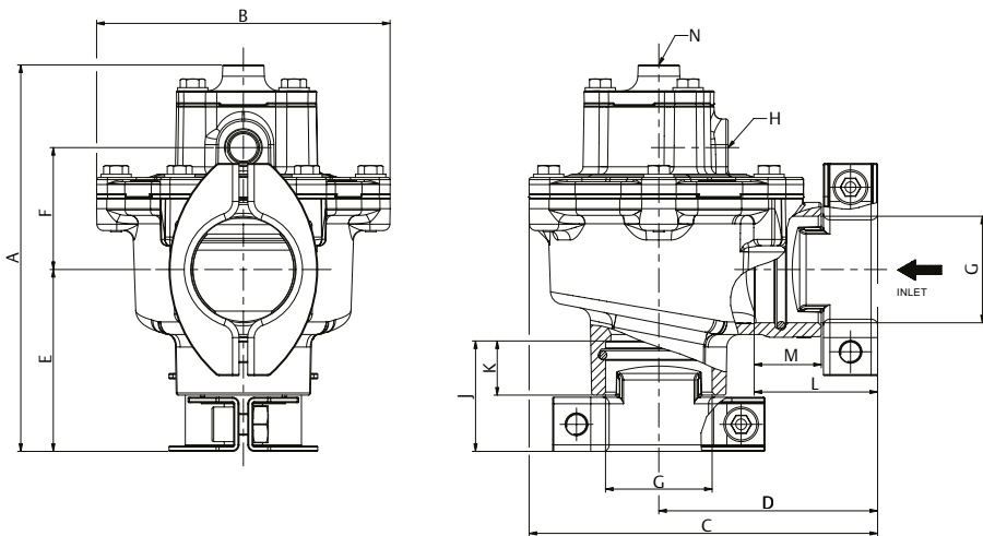
Рис. 6. 1 1/2", пневматический клапан
