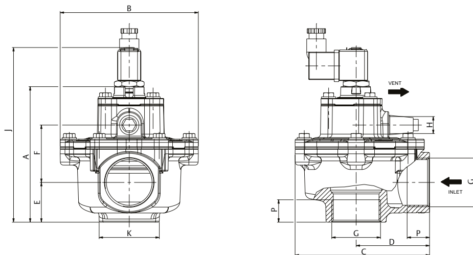
Рис. 7. 1 1/2", соленоидный клапан
