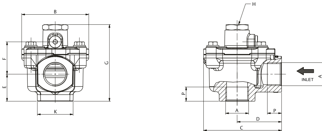
Рис. 4. Пневмоуправляемый импульсный клапан
