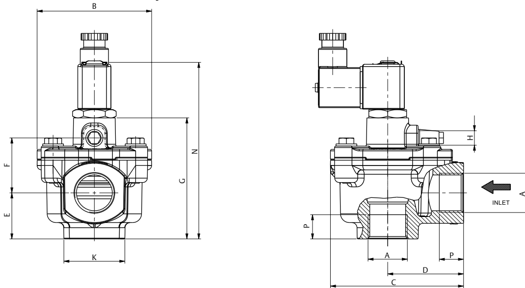
Рис. 3. Соленоидный импульсный клапан
