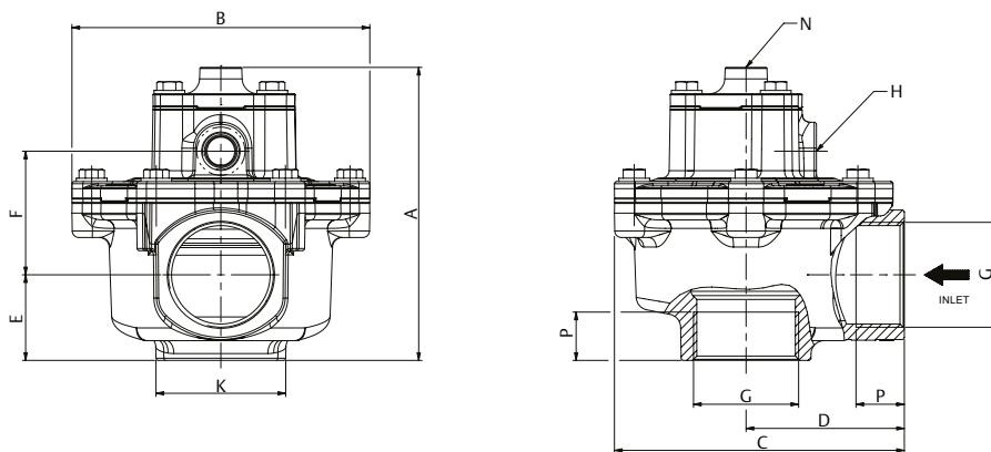
Рис. 8. 1 1/2", пневматический клапан
