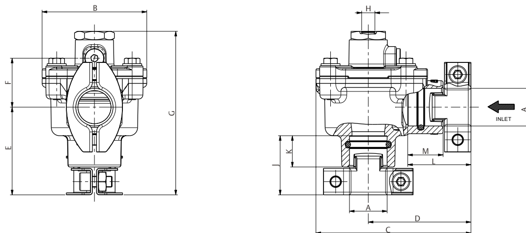
Рис. 2. Пневмоуправляемый импульсный клапан
