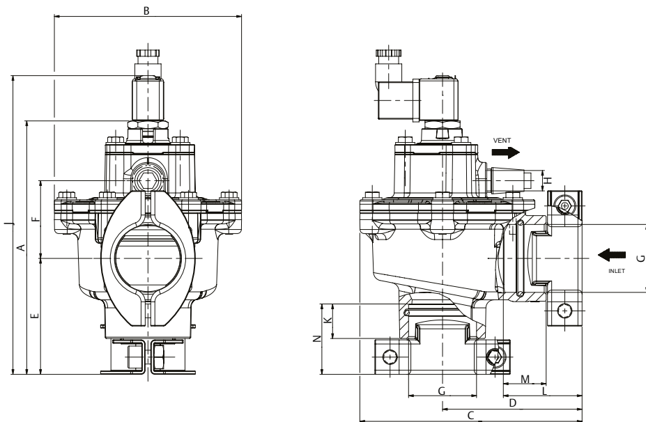
Рис. 5. 1 1/2", соленоидный клапан
