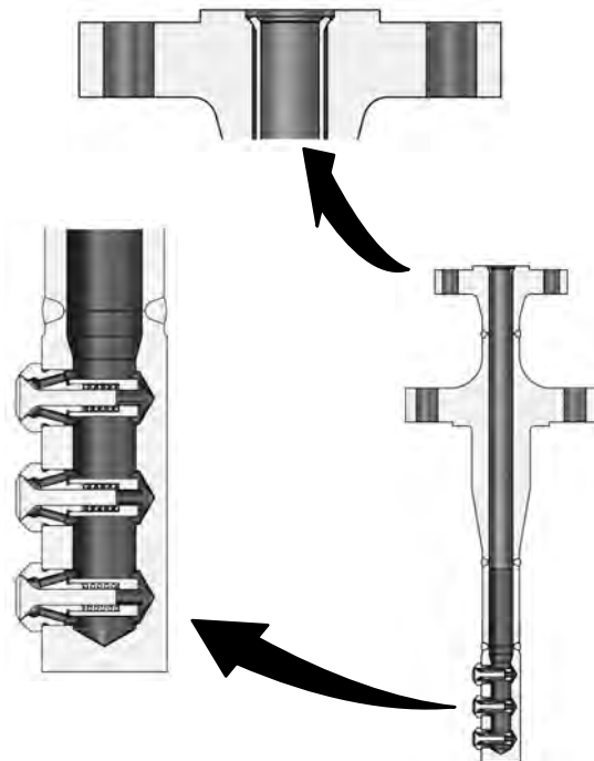
Рис. 3. Устройство пароохладителя DMA/AF-HTC компании Fisher
