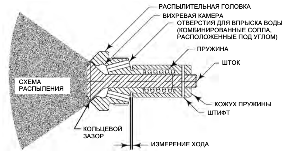
Рис. 5. Форсунка конструкции AF (DMA/AF и DMA/AF-НТС) компании Fisher
