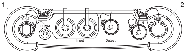
Рис. 7.13: Подключение датчиков к преобразователю
