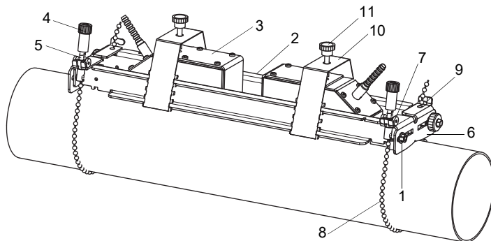
Рис. 6.11: Рельс Variofix с цепями
