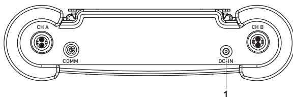
Рис. 7.19: Подключение блока питания к преобразователю FLUXUS *608**-F2
