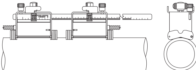
Рис. 6.10: Крепление датчиков с помощью магнитных монтажных башмаков
