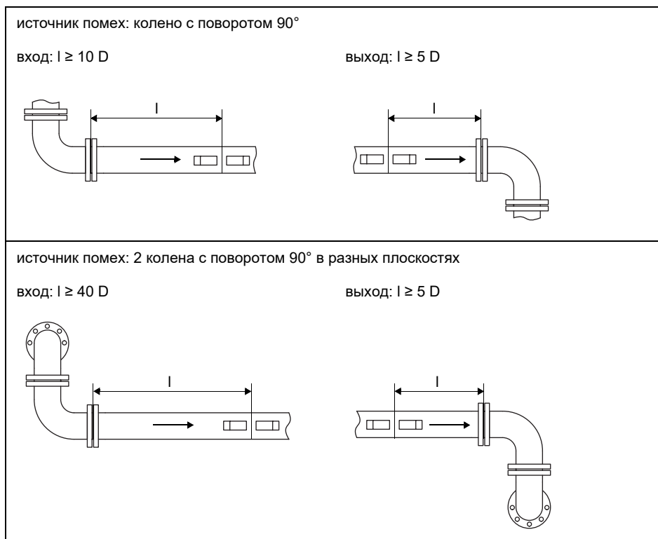
Таб. 3.1: Рекомендуемые расстояния от источников помех D – номинальный диаметр в месте измерения l – рекомендуемое расстояние между источником помех и позицией датчиков
