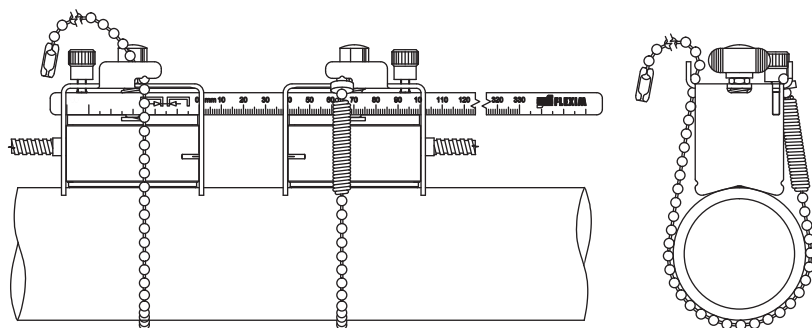
Рис. 6.9: Крепление датчиков с помощью монтажных башмаков и цепей
