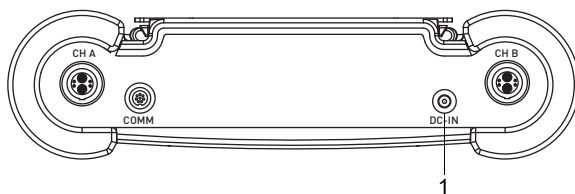
Рис. 7.22: Разъемы подключения преобразователя
