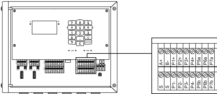
Рис. 7.16: Подключение выходов к преобразователю
