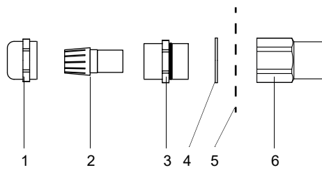
Рис. 7.25: Кабельный сальник
