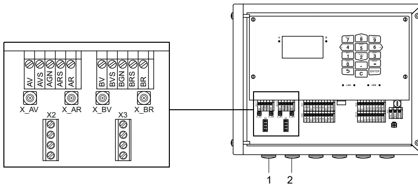
Рис. 7.1: Подключение датчиков к преобразователю
