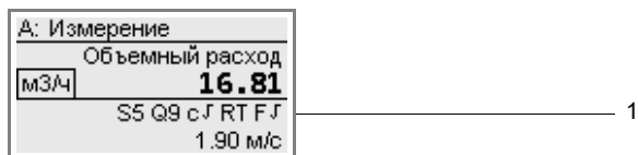
Рис. 10.5: Строка состояния
