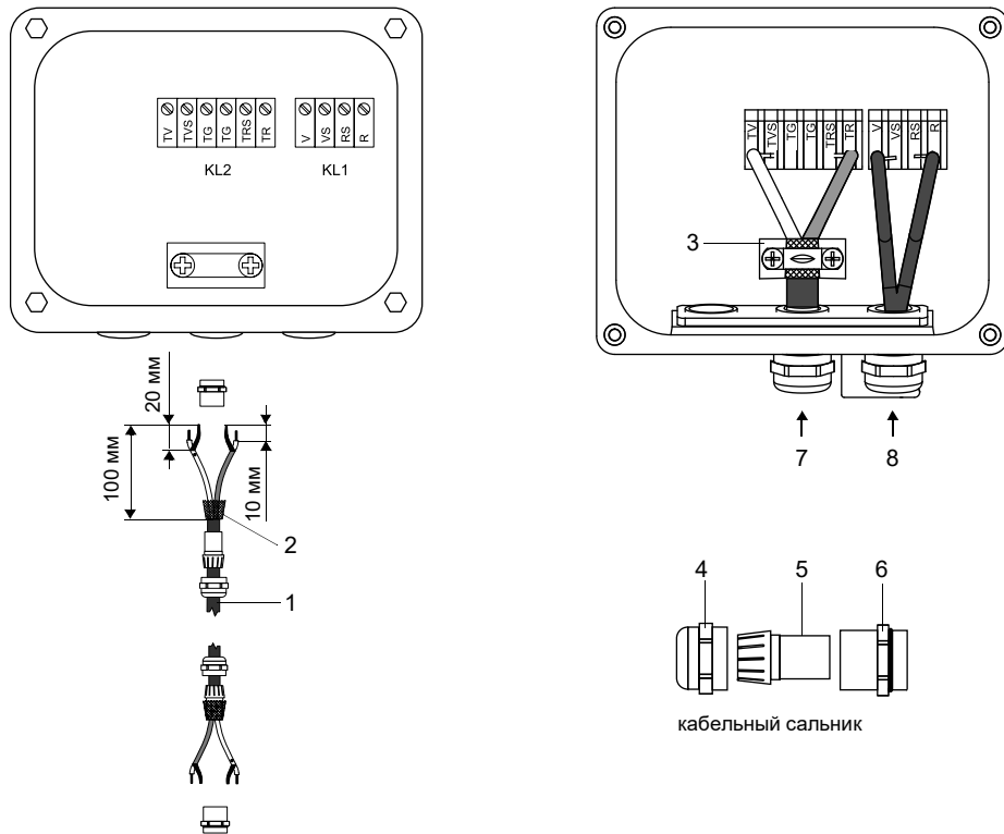
Рис. 8.10: Подключение удлинительного кабеля к соединительной коробке (с развязкой потенциалов)
