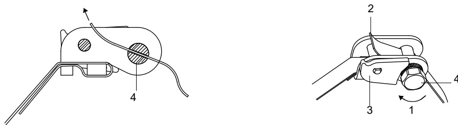
Рис. 7.54: Храповой замок со стальной лентой
