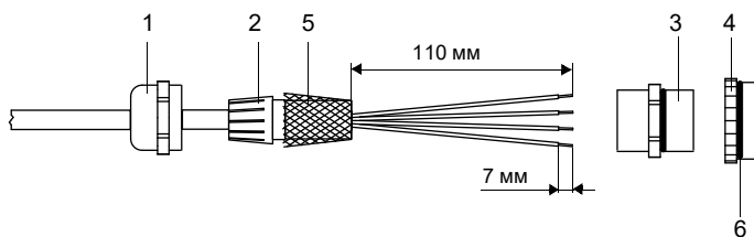
Рис. 8.19: Разделка датчика температуры
