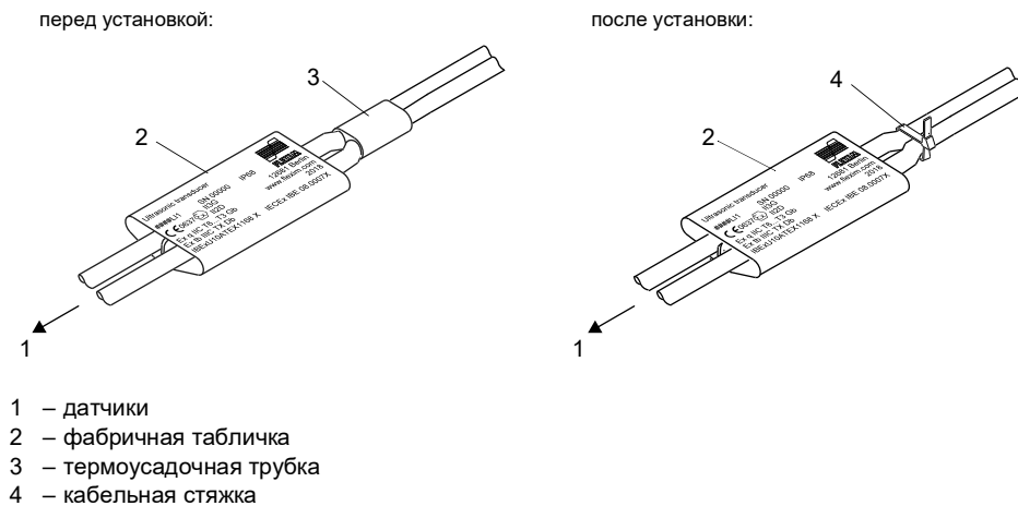
Рис. 7.10: Фабричная табличка на кабеле датчика
