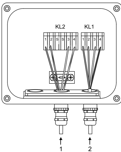
Рис. 8.22: Соединительная коробка
