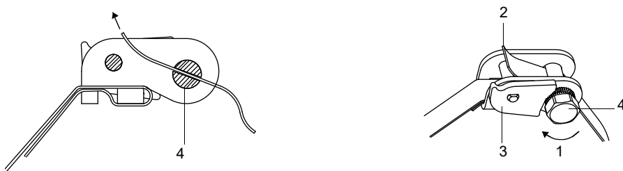
Рис. 7.47: Храповой замок со стальной лентой
