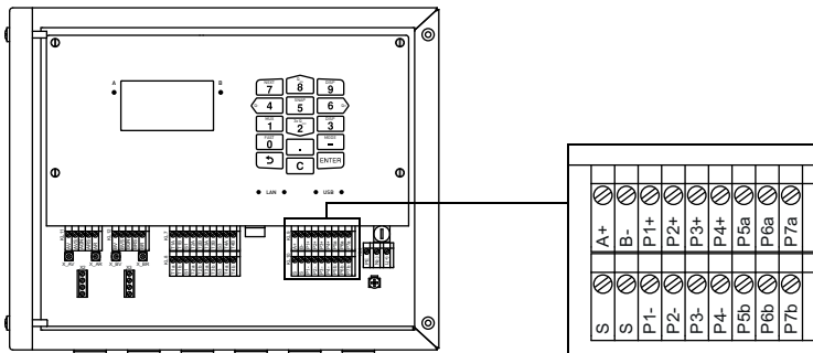
Рис. 8.16: Подключение выходов к преобразователю
