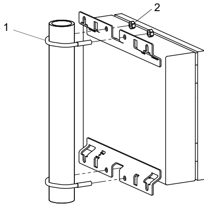
Рис. 7.6: Вид установки
