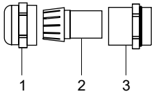
Рис. 8.15: Кабельный сальник для корпуса из алюминия
