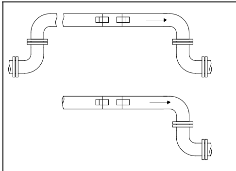
Рис. 4.13: непригодное размещение датчиков
