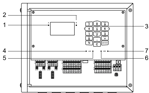
Рис. 9.1: Панель управления преобразователя
