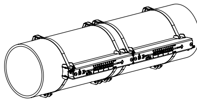
Рис. 7.12: Крепление датчика Variofix L (режим отражения)
