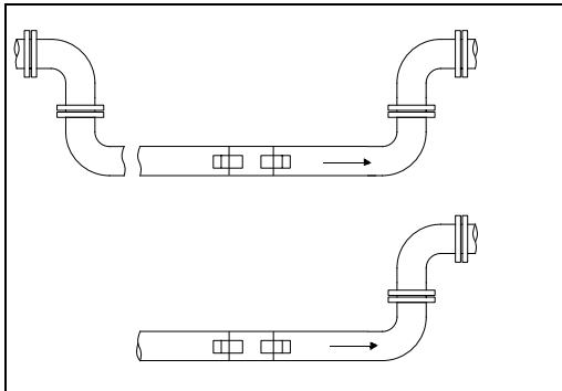
Рис. 4.12: Рекомендуемое размещение датчиков
