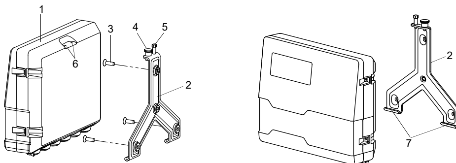
Рис. 7.5: Вид установки
