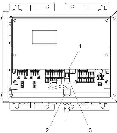
Рис. 8.24: Подключение кабеля ЛВС
