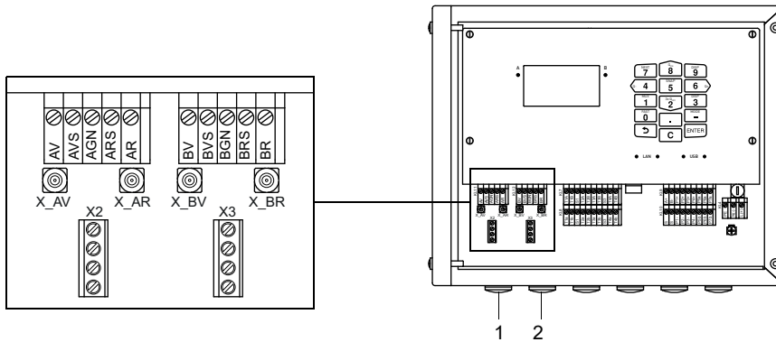
Рис. 8.1: Подключение датчиков к преобразователю
