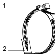
Рис. 7.52: Стальная лента с быстросъемным замком и металлической пружиной
