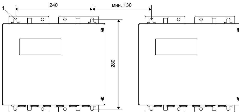
Рис. 7.3: Преобразователь (размеры в мм)
