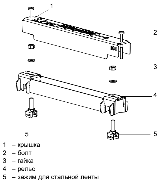
Рис. 7.13: Разборка крепления датчика Variofix L
