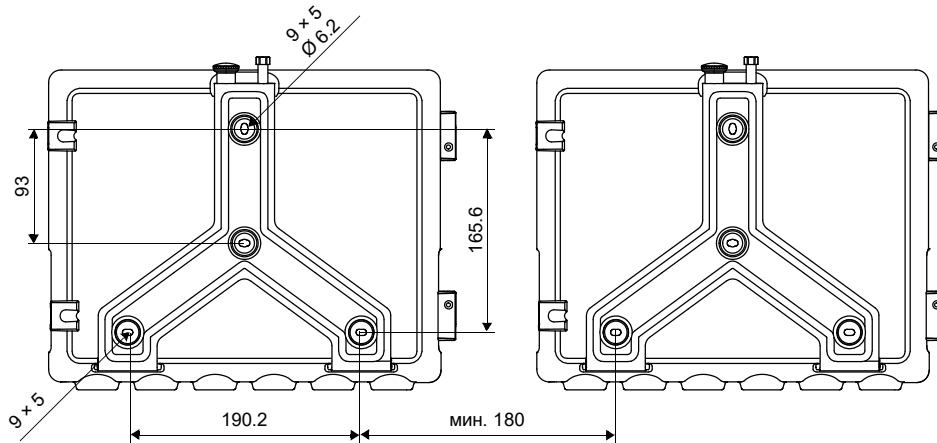
Рис. 7.4: Преобразователь (размеры в мм)
