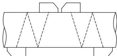
Рис. 4.4: Режим диагональ с 2-мя лучами и 3-мя проходами звука
