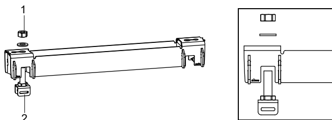
Рис. 7.23: Рельс с зажимом для стальной ленты
