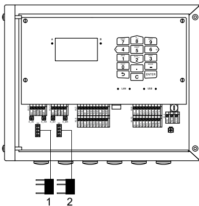
Рис. 8.11: Память SENSPROM
