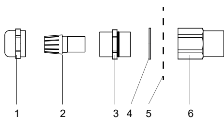
Рис. 8.14: Кабельный сальник для корпуса из нержавеющей стали
