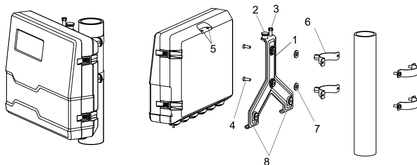
Рис. 7.7: Вид установки
