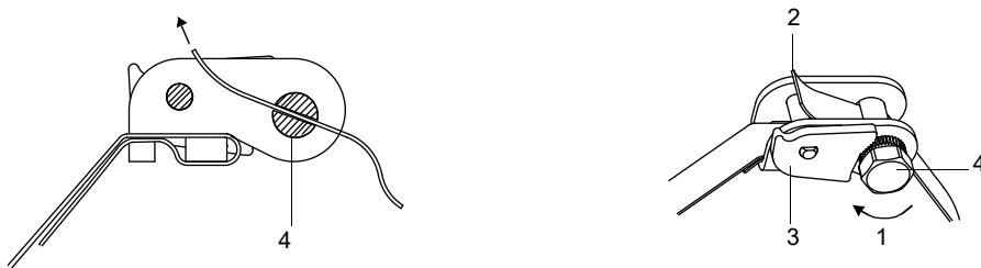
Рис. 7.22: Храповой замок со стальной лентой
