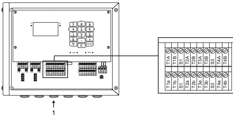
Рис. 8.18: Подключение датчиков температуры к преобразователю
