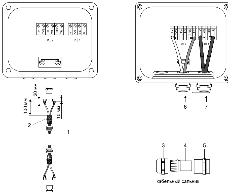
Рис. 8.9: Подключение удлинительного кабеля к соединительной коробке (без развязки потенциалов)
