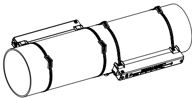
Рис. 7.11: Крепление датчика Variofix L (режим диагональ)
