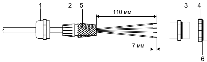
Рис. 8.21: Разделка удлинительного кабеля
