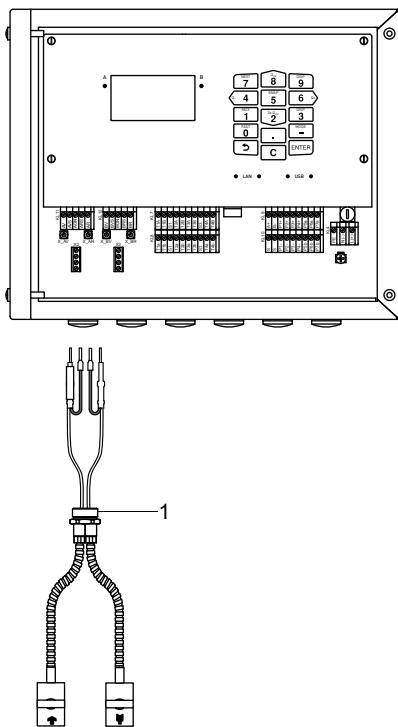
Рис. 8.4: Подключение кабеля датчика с кабелепроводом из нержавеющей стали и неизолированными концами к преобразователю
