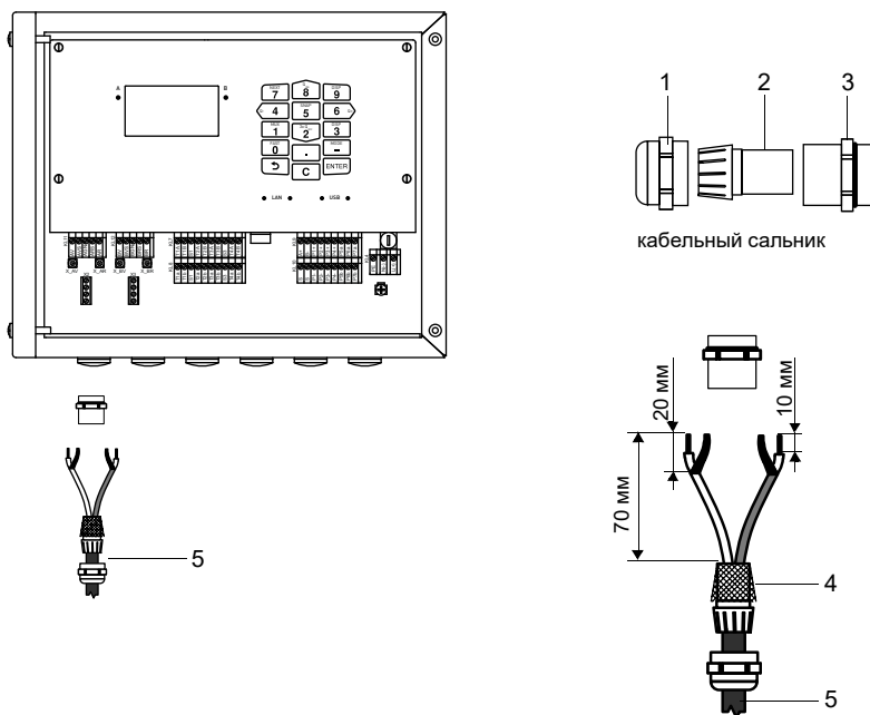
Рис. 8.5: Подключение удлинительного кабеля к преобразователю
