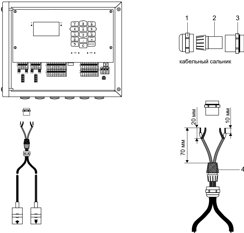
Рис. 8.3: Подключение кабеля датчика с пластмассовой изоляцией и неизолированными концами к преобразователю
