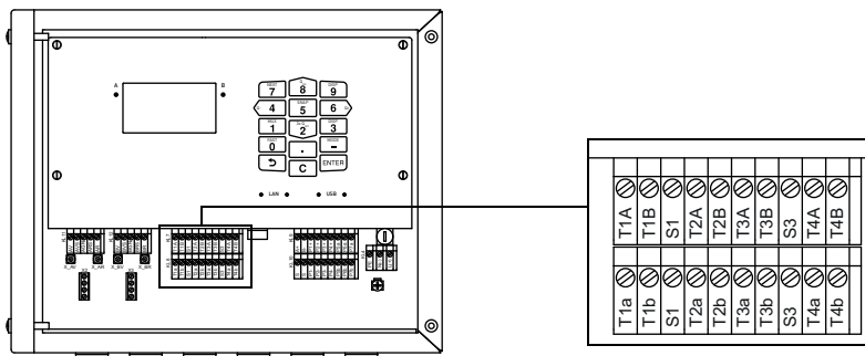
Рис. 8.17: Подключение входов к преобразователю
