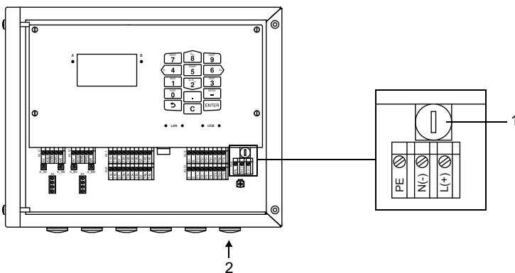
Рис. 8.13: Подключение питания напряжения к преобразователю
