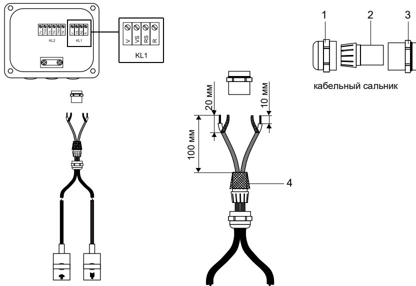
Рис. 8.7: Подключение кабеля датчика с пластмассовой изоляцией и неизолированными концами
