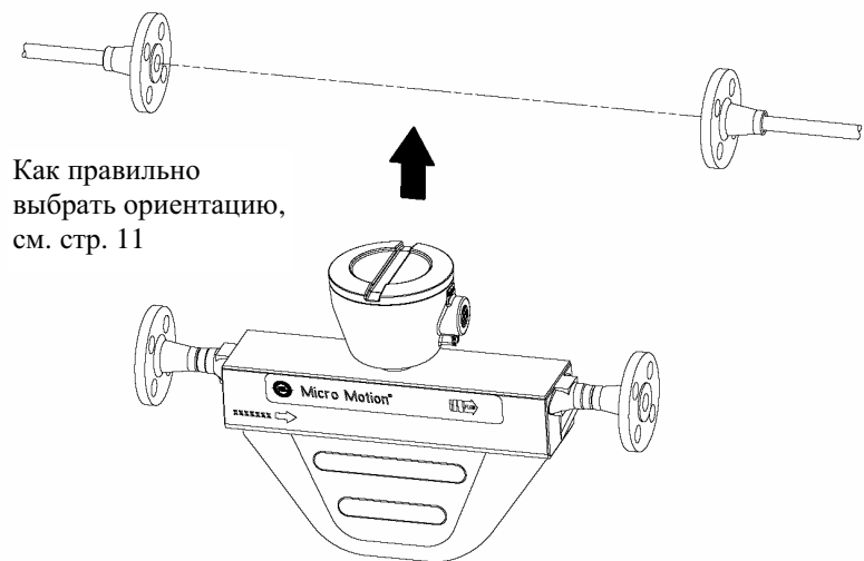
Рисунок 4-1. Монтаж сенсора
