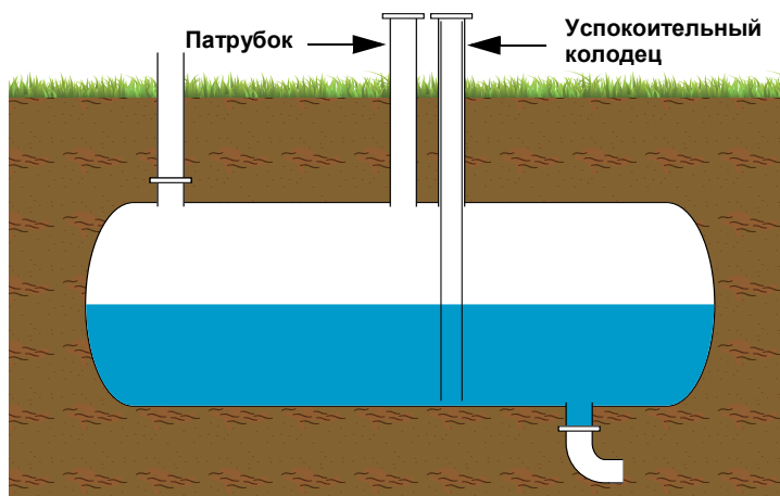
Рис. 1. Подземный резервуар с высоким патрубком и успокоительным колодцем
