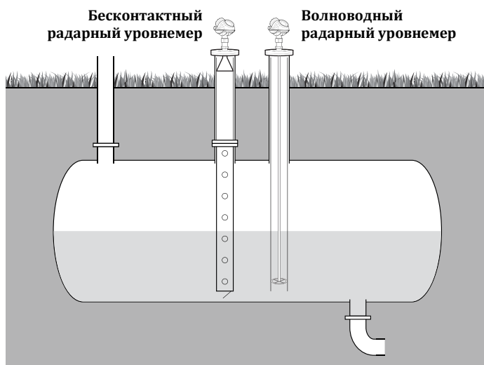
Рис. 2. Патрубок, реконструированный при помощи успокоительного колодца
