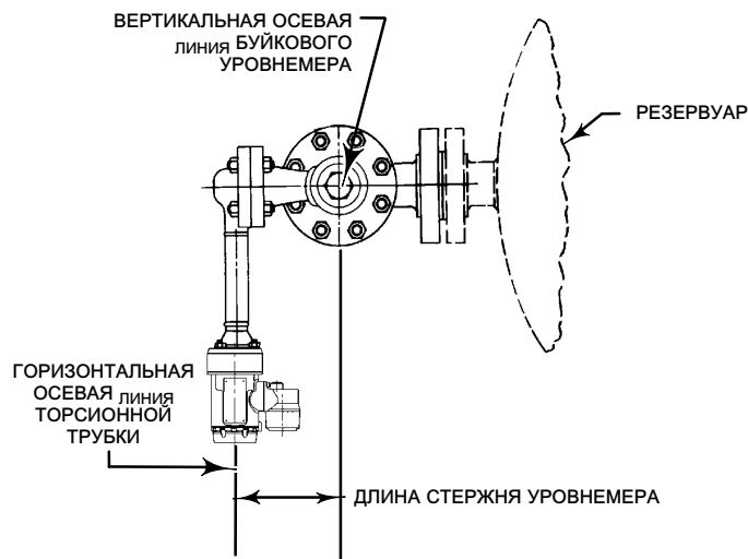
Рис. 12. Определение длины стержня привода путем проведения внешних измерений
