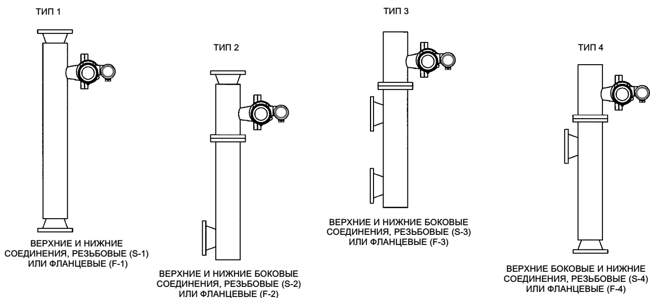
Рис. 20. Различные типы уравнительных соединений
