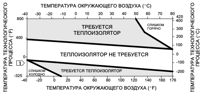
Рис. 7. Основные принципы применения дополнительного узла теплоизолятора
