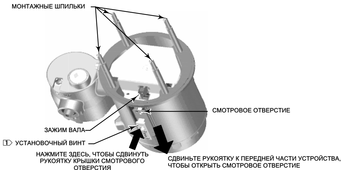
Рис. 2. Отсек подключения датчика (без переходного кольца)
