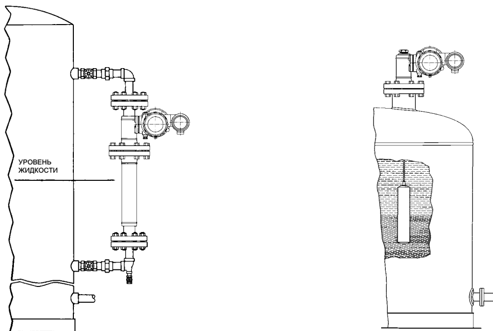
СТАНДАРТНЫЙ МОНТАЖ ДАТЧИКА С КАМЕРОЙ
