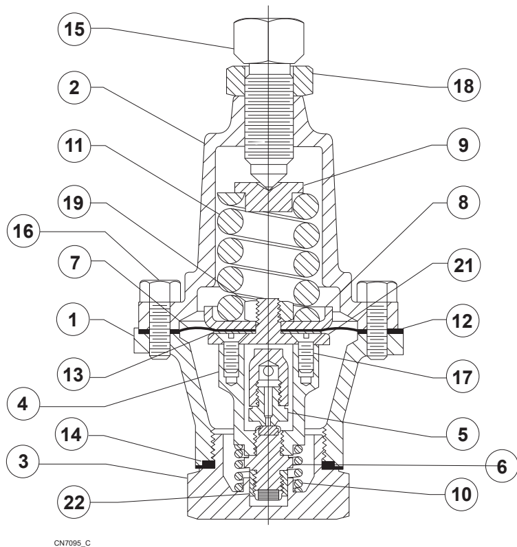
Figur 4. Type 1301G Højtryksregulator
