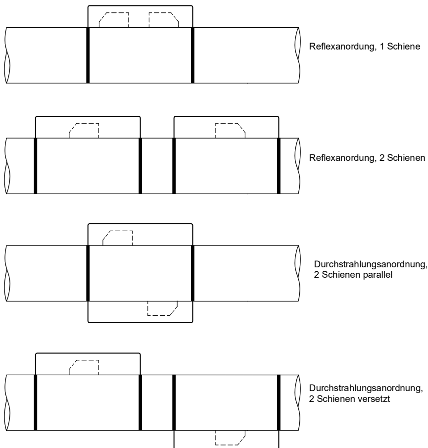
Abb. 6.6: Anordnung der Sensoren in Montage-Schienen
