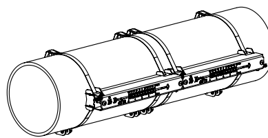
Abb. 6.8: Sensorbefestigung Variofix L (Reflexanordnung)
