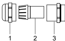
Abb. 7.12: Kabelverschraubung
