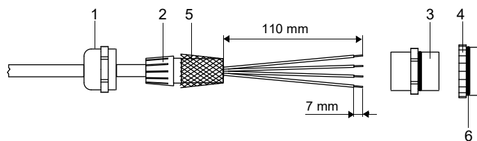
Abb. 7.17: Konfektionierung des Verlängerungskabels
