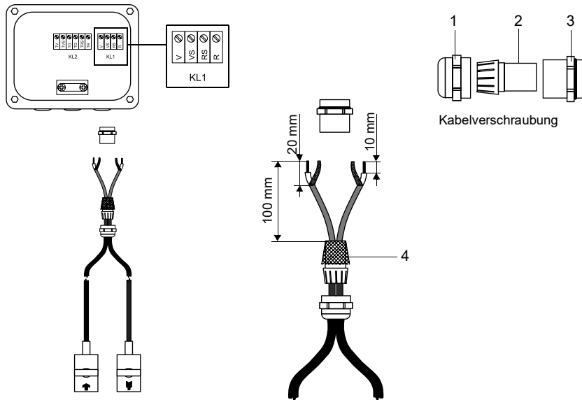
Abb. 7.6: Anschluss des Sensorkabels mit Kunststoffkabelmantel und abisolierten Kabelenden
