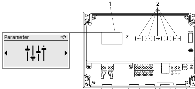
Abb. 4.2: Bedienungsfeld des Messumformers
