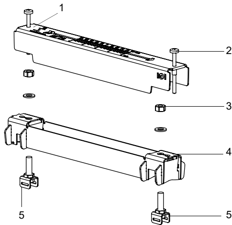
Abb. 6.9: Demontage von Variofix L
