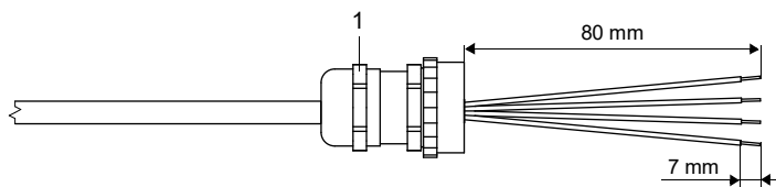
Abb. 7.19: Konfektionierung
