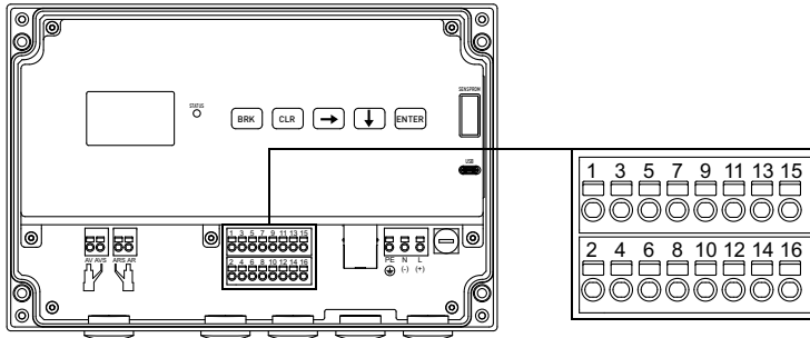
Abb. 7.15: Anschluss der Temperaturfühler am Messumformer
