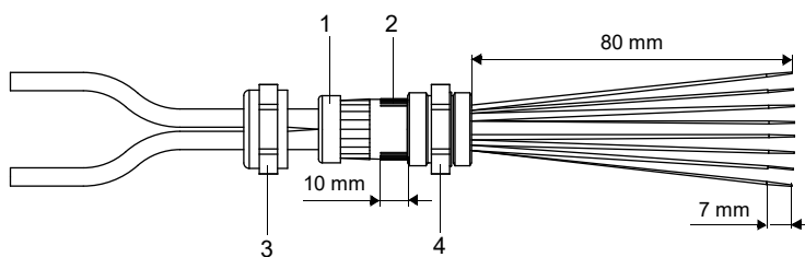
Abb. 7.21: Kabelverschraubung und Konfektionierung
