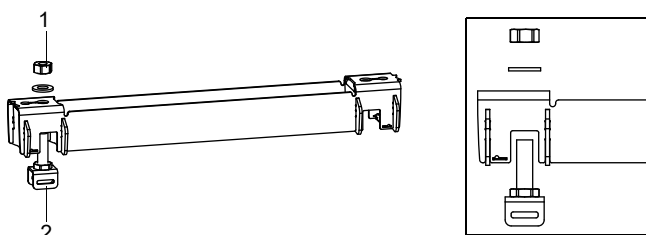
Abb. 6.19: Schiene mit Spannbandklammer
