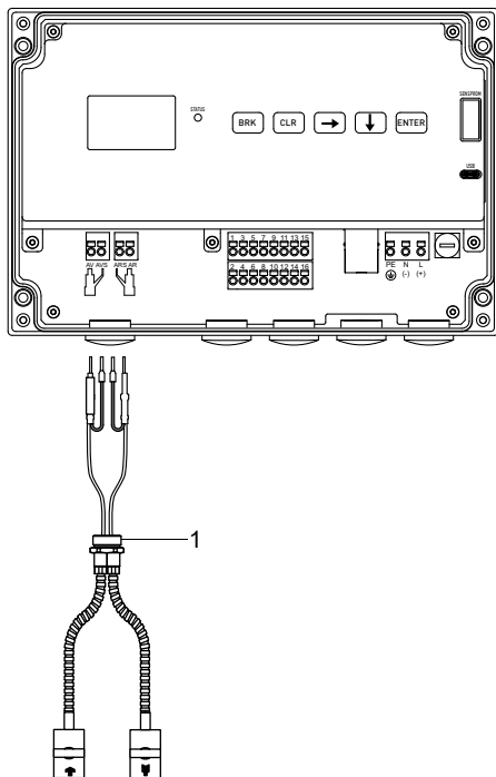
Abb. 7.4: Anschluss des Sensorkabels mit Edelstahlmantelung und abisolierten Kabelenden an den Messumformer
