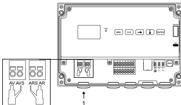
1 – Anschluss der Sensoren
