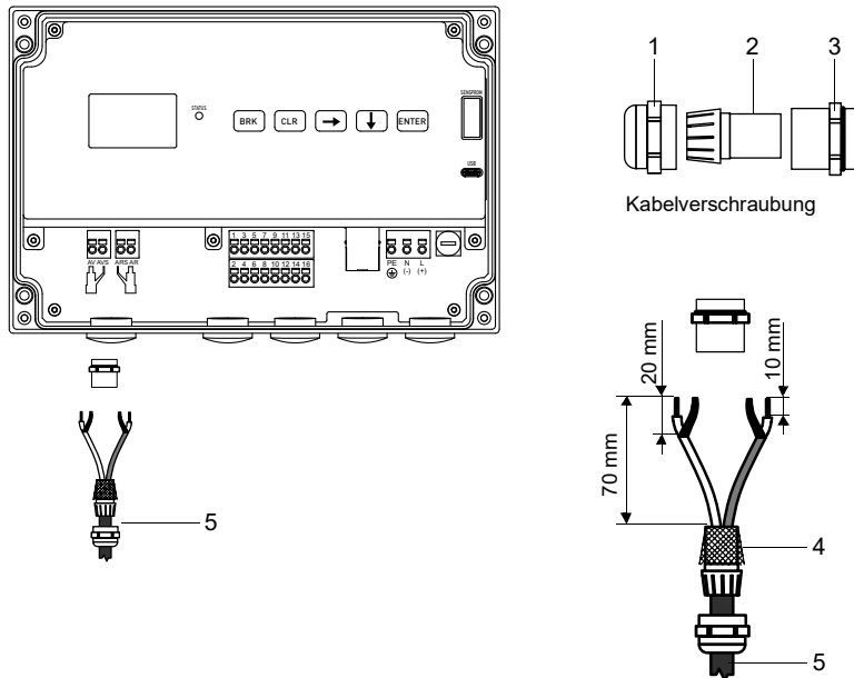
Abb. 7.5: Anschluss des Verlängerungskabels an den Messumformer
