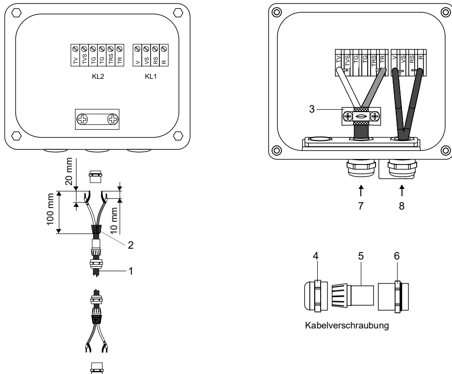
Abb. 7.9: Anschluss des Verlängerungskabels an das Klemmgehäuse (mit Potentialtrennung)
