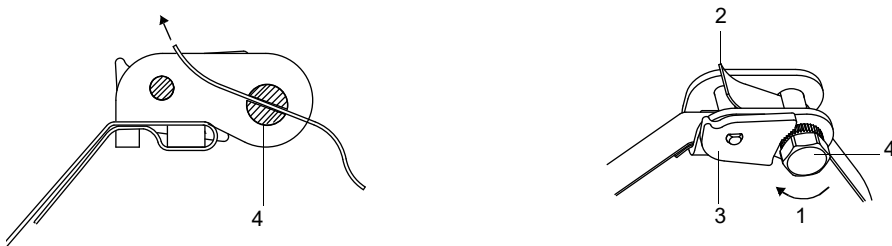
Abb. 6.18: Ratschenschloss mit Spannband
