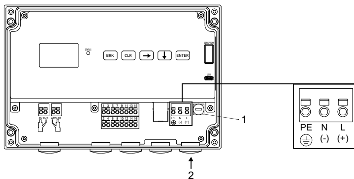
Abb. 7.11: Anschluss der Spannungsversorgung am Messumformer
