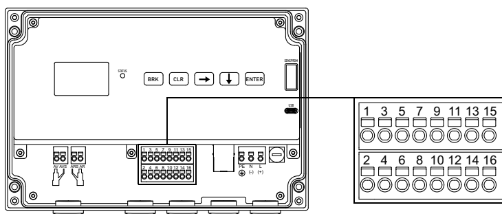
Abb. 7.14: Anschluss der Ausgänge am Messumformer
