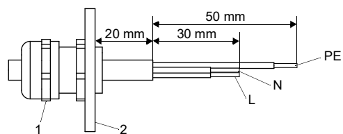
Abb. 7.13: Konfektionierung des Spannungsversorgungskabels
