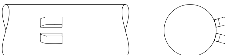
Abb. 3.5: Messanordnung im NoiseTrek-Parallelstrahl-Modus
