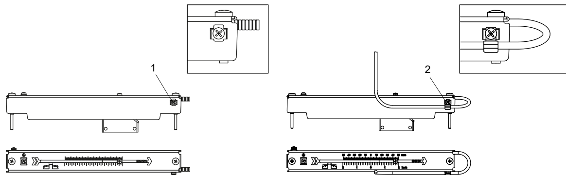
Abb. 6.29: Fixieren der Sensorkabel
