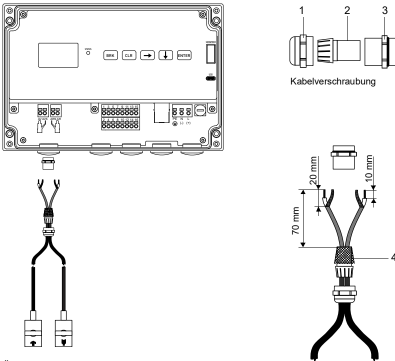
Abb. 7.3: Anschluss des Sensorkabels mit Kunststoffkabelmantel und abisolierten Kabelenden an den Messumformer
