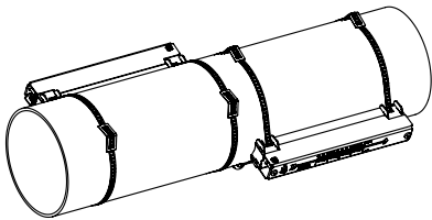
Abb. 6.7: Sensorbefestigung Variofix L (Durchstrahlungsanordnung)
