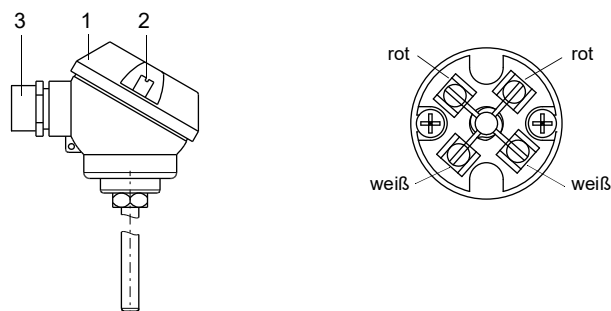
Abb. 7.20: Anschlusskopf des Inline-Temperaturfühlers
