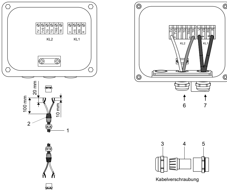
Abb. 7.8: Anschluss des Verlängerungskabels an das Klemmengehäuse (ohne Potentialtrennung)
