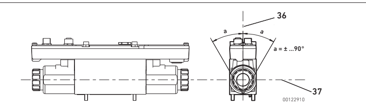
fig 3: Monteringsläge
