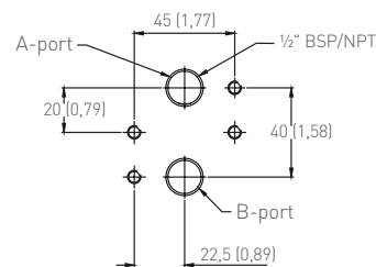
Lufttilkobling, størrelsen 240
