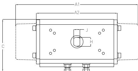
Toppvisningsmodell 002 – 020
