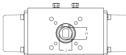
Toppvisningsmodell 032 – 240
