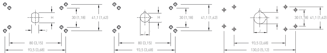
Boringsstørrelser til topmontering 002 - 020
