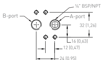
Storlekar luftanslutning 002 - 052
