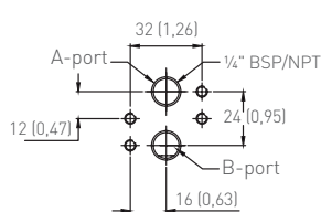
Storlekar luftanslutning 085 - 140
