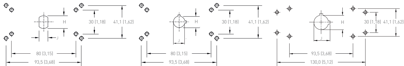
Övre borrhingsstorlekar för montering 002 - 020
