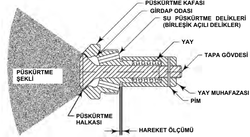
Şekil 5. Fisher AF Enjektör (DMA/AF ve DMA/AF-HTC)
