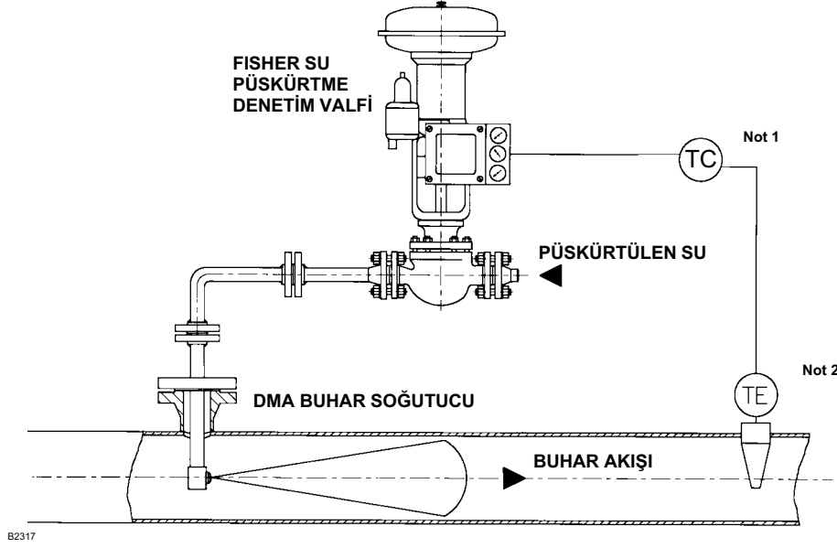
Şekil 4. Fisher DMA, DMA/AF veya DMA/AF-HTC Buhar Soğutucularının Tipik Kurulum Düzeni
