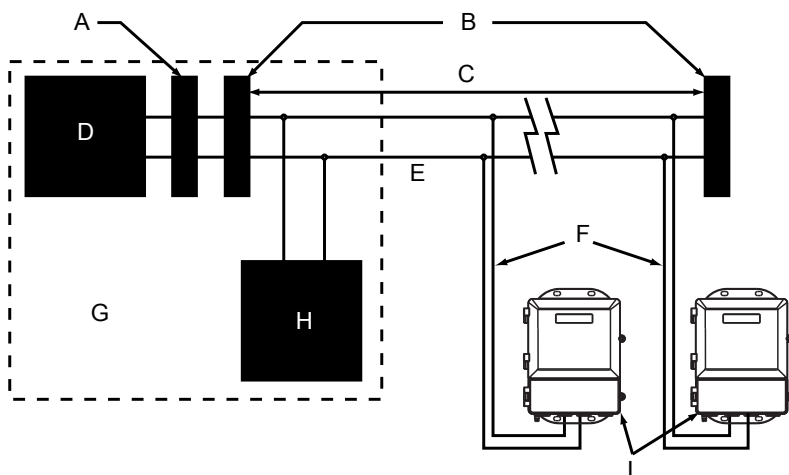
Figura 5-12: Collegamenti di alimentazione
