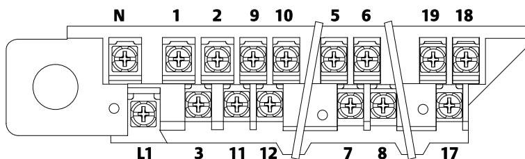
Figura 5-8: Morsettiere
