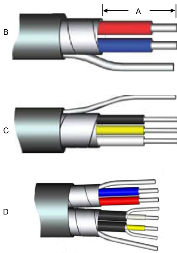
Figura 5-4: Estremità dei cavi
