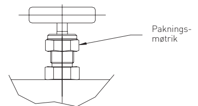
H1- \frac{3}{8} " OG \frac{5}{8} " ÅBNING, H5 PTFE og Graphite pakningstyper
