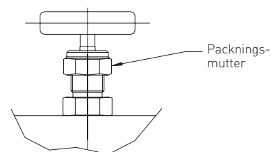
H1 - ANSLUTNINGSDIAM. 3/8" OCH 1/2", H5 - P.T.F.E.- och grafitpackningar
