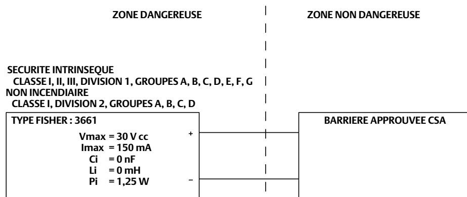
Figure 1. Schéma de boucle (Schéma GE28591)
