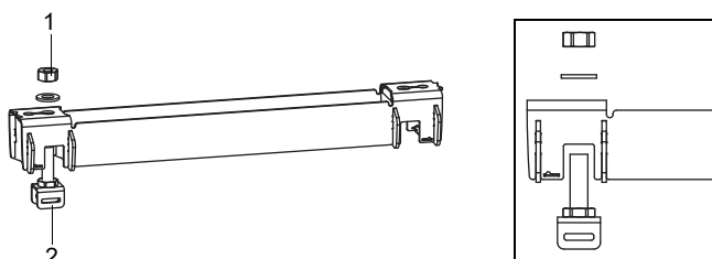
Fig. 6.20: Riel con sujetador para cinta de sujeción
