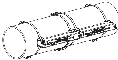
Fig. 6.9: Porta-transductor Variofix L (configuración en modo de reflexión)
