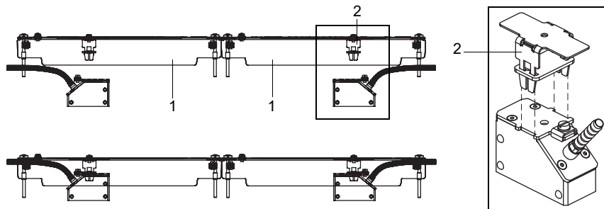
Fig. 6.28: Montaje de los transductores en las cubiertas
