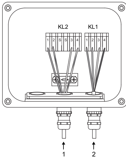
Fig. 7.19: Caja de bornes
