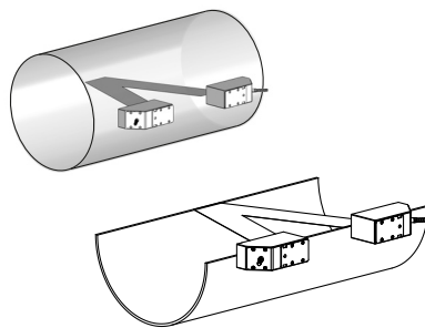
Fig. 3.8: 2 trayectorias de sonido en un plano
