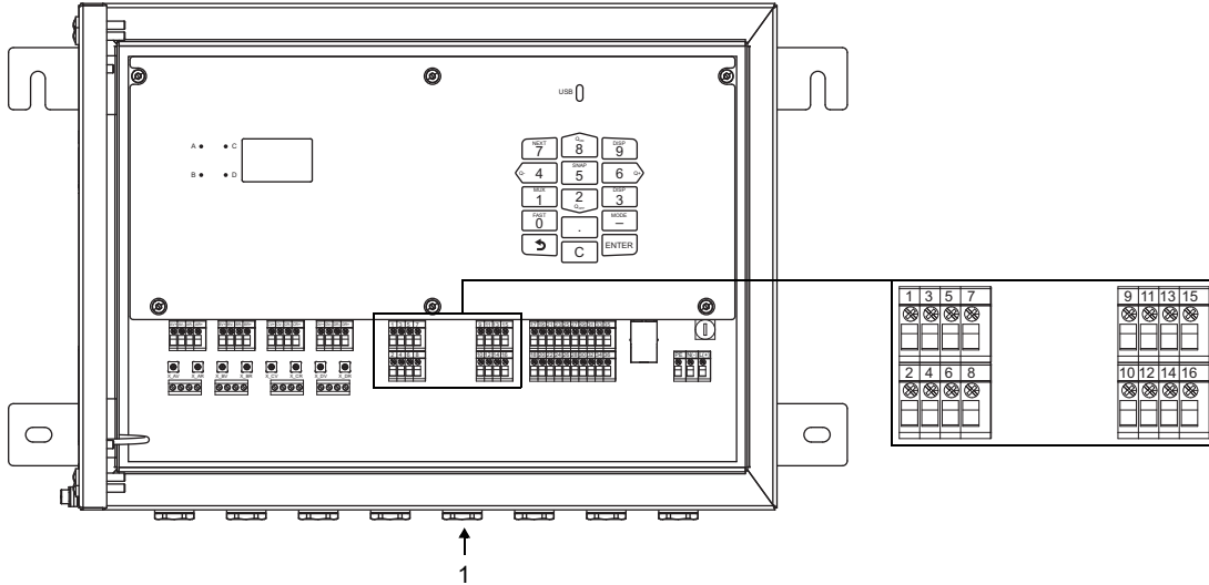
Fig. 7.16: Conexión del sensor de temperatura en el transmisor
