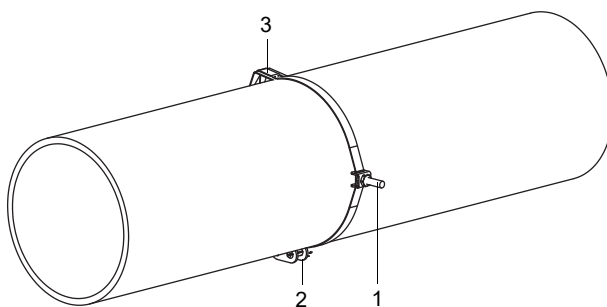
Fig. 6.14: Cinta de sujeción con sujetador y resorte metálico en la tubería
