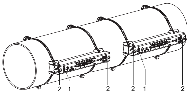
Fig. 6.31: Variofix L con transductor en la tubería
