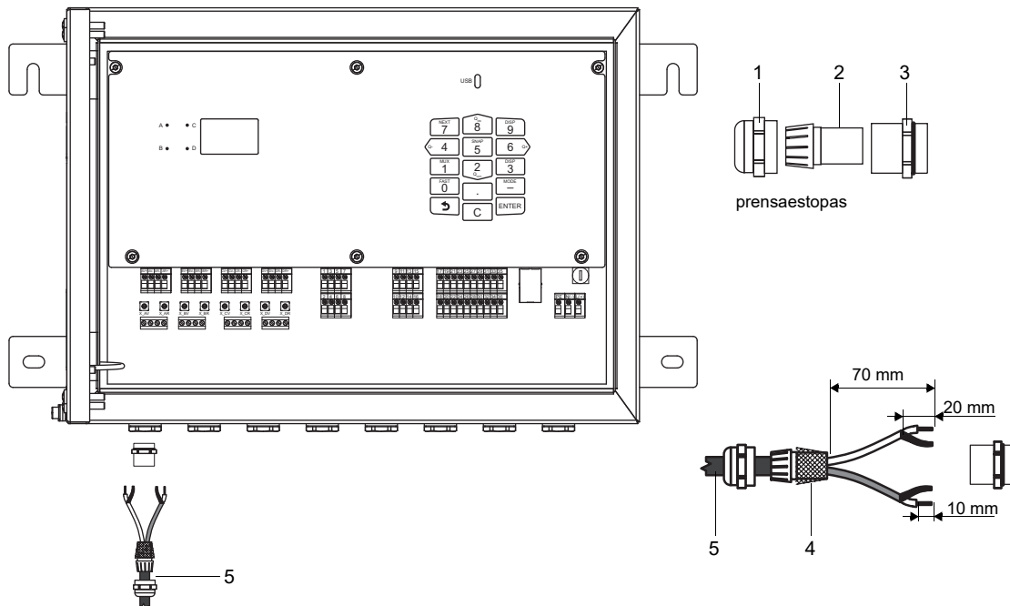
Fig. 7.5: Conexión de la extensión en el transmisor
