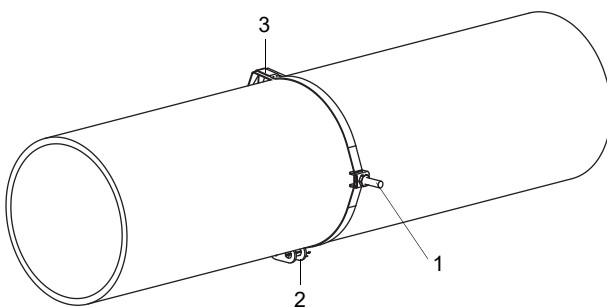
Fig. 6.39: Cinta de sujeción con sujetador y resorte metálico en el tubo
