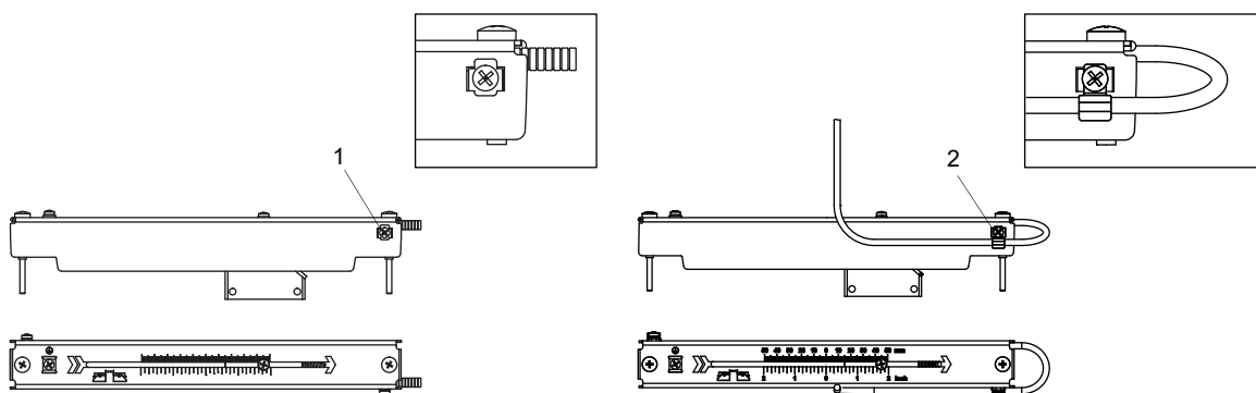
Fig. 6.30: Fijación del cable del transductor
