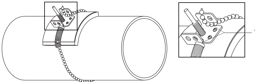
Fig. 6.63: Sensor de temperatura en la tubería
