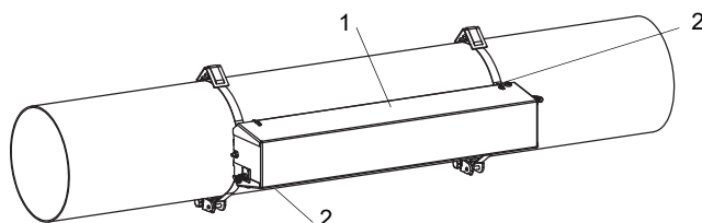
Fig. 6.55: Variofix C con transductores en la tubería
