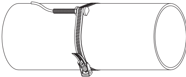
Fig. 6.59: Sensor de temperatura en la tubería
