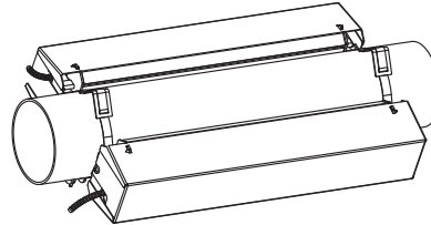
Fig. 6.33: Porta-transductores Variofix C (configuración en modo diagonal)
