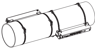
Fig. 6.8: Porta-transductor Variofix L (configuración en modo diagonal)
