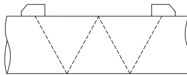
Fig. 3.6: Configuración en modo de reflexión con 1 haz y 4 trayectorias de sonido
