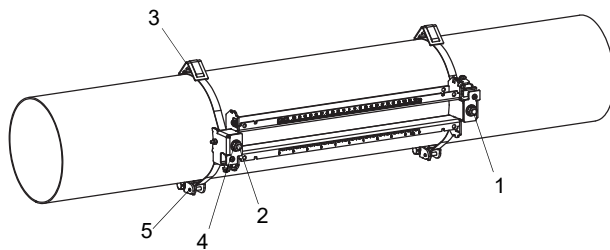
Fig. 6.47: Riel en la tubería
