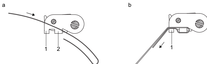
Fig. 6.38: Cierre de trinquete con cinta de sujeción
