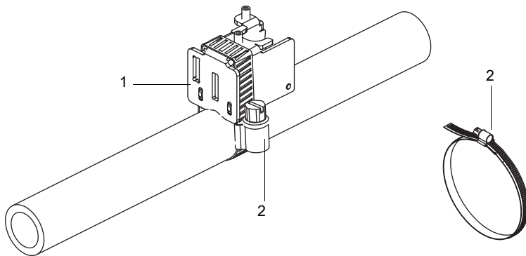
Fig. 6.57: Transductor en dispositivo de montaje, montado con cinta de sujeción y tensor
