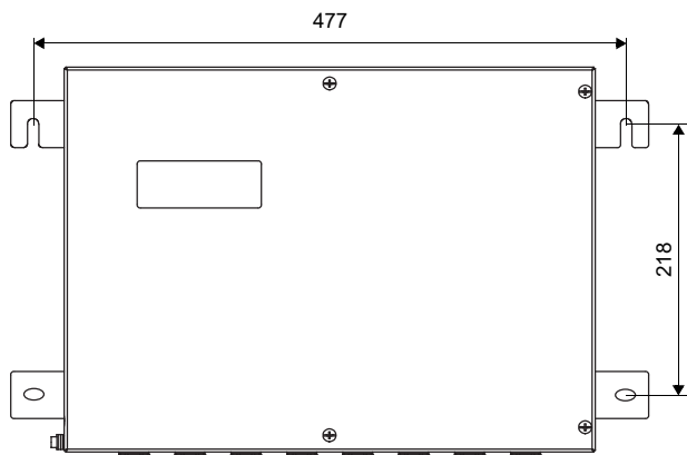
Fig. 6.2: Transmisor (dimensiones en mm)
