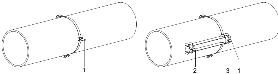
Fig. 6.21: Riel montado en un lado de la tubería
