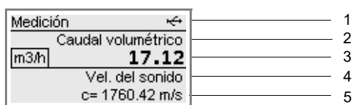
Fig. 9.2: Visualización de los valores de medición
