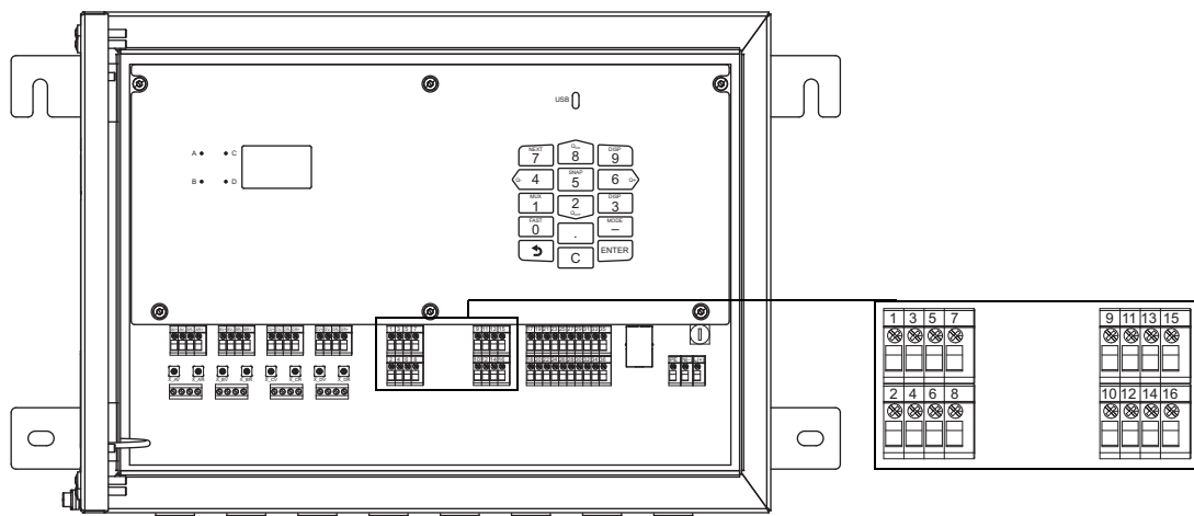
Fig. 7.15: Conexión de las entradas al transmisor
