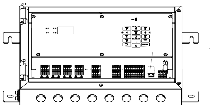
Fig. 7.21: Conexión del cable LAN
