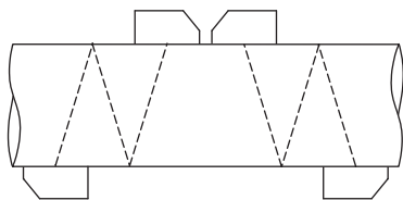
Fig. 3.5: Configuración en modo diagonal con 2 haces y 3 trayectorias de sonido
