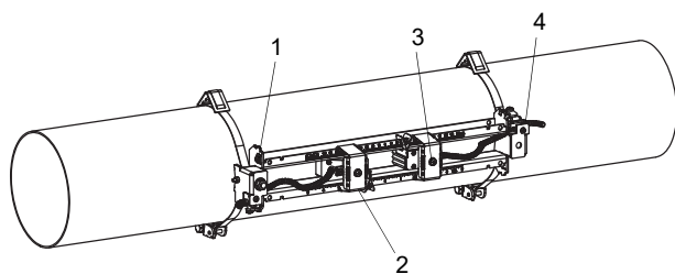
Fig. 6.54: Transductores en el riel
