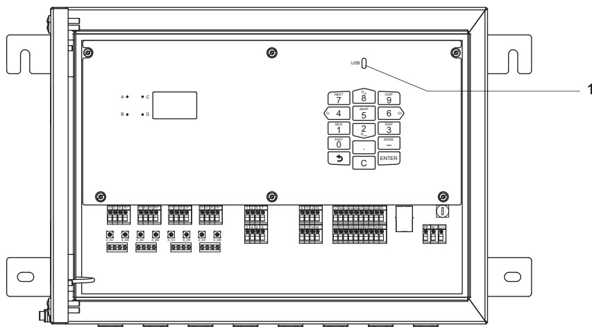
Fig. 7.20: Conexión del cable USB
