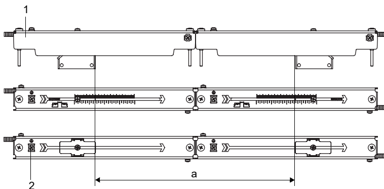
Fig. 6.29: Ajuste de la distancia entre transductores
