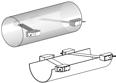
Fig. 3.7: 2 haces en un plano
