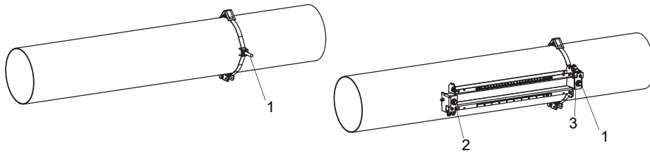
Fig. 6.46: Riel montado en un lado de la tubería
