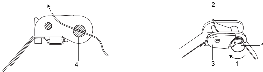
Fig. 6.19: Cierre de trinquete con cinta de sujeción
