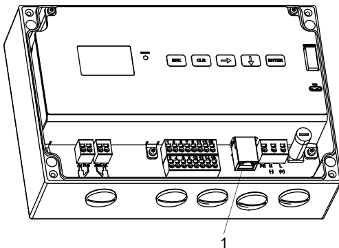
Fig. 7.25: Conexión del cable LAN
