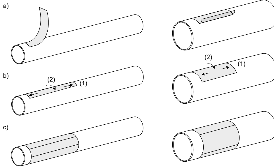
Fig. 6.8: Fijación de las esteras de amortiguamiento
