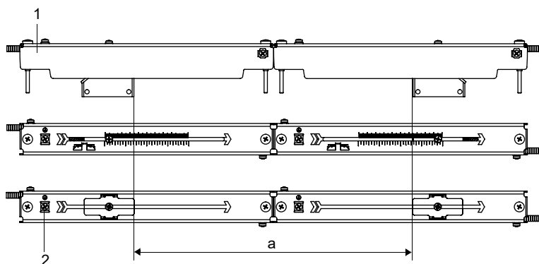
Fig. 6.33: Ajuste de la distancia entre transductores
