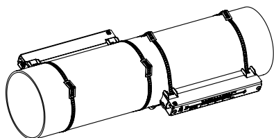
Fig. 6.12: Porta-transductor Variofix L (configuración en modo diagonal)
