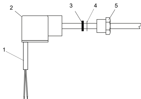
Fig. 7.15: Montaje del cable
