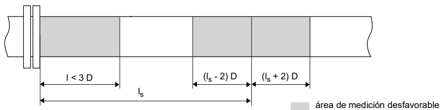
Fig. 3.10: Puntos de medición a evitar
