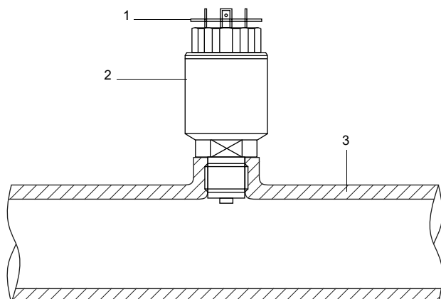
Fig. 6.42: Transmisor de presión montado
