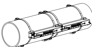
Fig. 6.13: Porta-transductor Variofix L (configuración en modo de reflexión)
