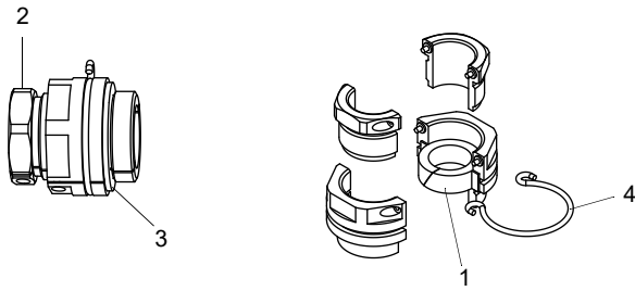
Fig. 7.26: Prensaestopas partido
