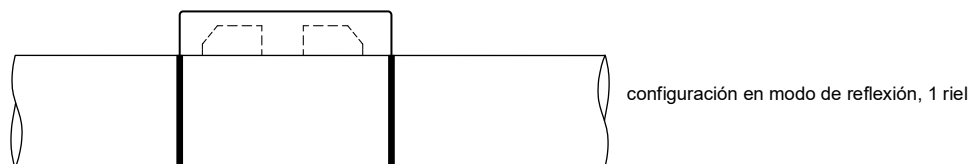
Fig. 6.11: Configuración de los transductores en rieles de montaje
