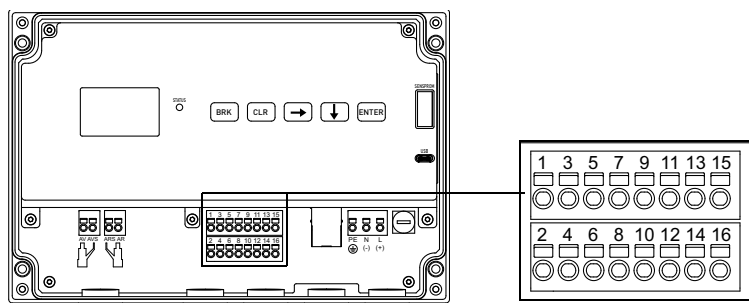
Fig. 7.11: Conexión de las entradas al transmisor
