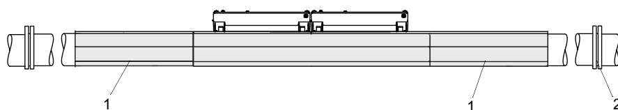
Fig. 6.6: Esteras de amortiguamiento para el transductor y la tubería en configuración en modo de reflexión
