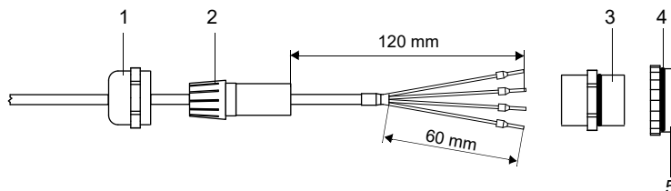
Fig. 7.13: Confección del sensor de temperatura
