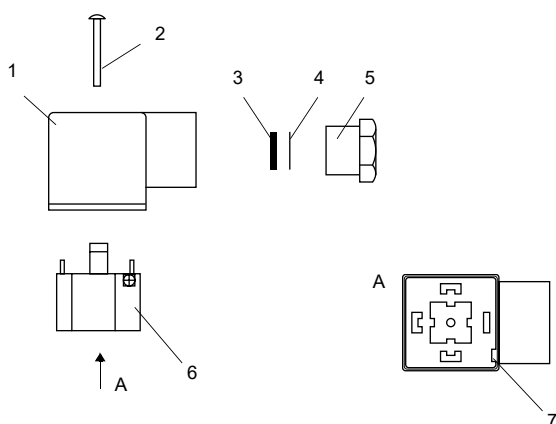
Fig. 7.14: Conector desmontado
