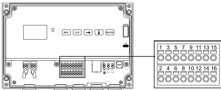
Fig. 7.21: Conexión de las entradas al transmisor
