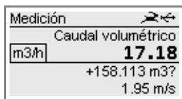
Fig. 4.4: Visualización del estado (línea 1)
