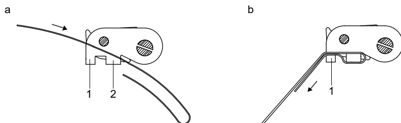
Fig. 6.17: Cierre de trinquete con cinta de sujeción
