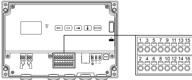
Fig. 7.12: Conexión del sensor de temperatura en el transmisor
