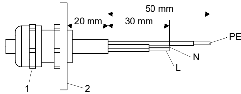
Fig. 7.9: Confección del cable de alimentación
