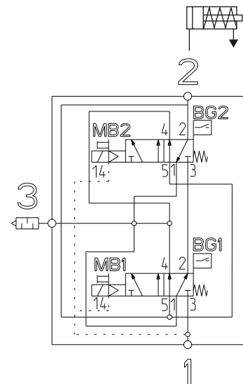
Anwendungsbeispiel | Exemple d'application | Application example | Esempio di applicazione | Ejemplo de aplicación | Användningsexempel
