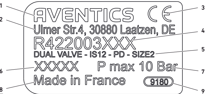
Typenschild | Plaque signalétique | Name plate | Targhetta dati | Placa de características | Typskylt 1: Firmenname | nom de la société | Company name | nome azienda | Nombre de la empresa | Tillverkarnamn 2: Firmenadresse | adresse de la société | Company address | indirizzo azienda | Dirección de la empresa | Tillverkarens adress 3: CE-Kennzeichnung | marquage CE | CE mark | marchio CE | Marcado CE | CE-märkning 4: Materialnummer | référence | Material number | codice | Número de material | Materialnummer 5: Typenbezeichnung | Désignation | Type designation | denominazione del tipo | Denominación de tipo | Typbeteckning 6: Fertigungsdatum | date de fabrication | Production date | data di produzione | Fecha de fabricación | Tillverkningsdatum 7: Maximaldruck | pression maximale | Maximum pressure | pressione massima | Presión máxima | Maximallt tryck 8: Herstellungsland | pays de fabrication | Country of manufacture | paese di produzione | País de fabricación | Tillverkningsland 9: Verantwortliches Werk | usine responsable | Responsible plant | stabilimento responsabile | Fábrica responsable | Ansvarig fabrik
