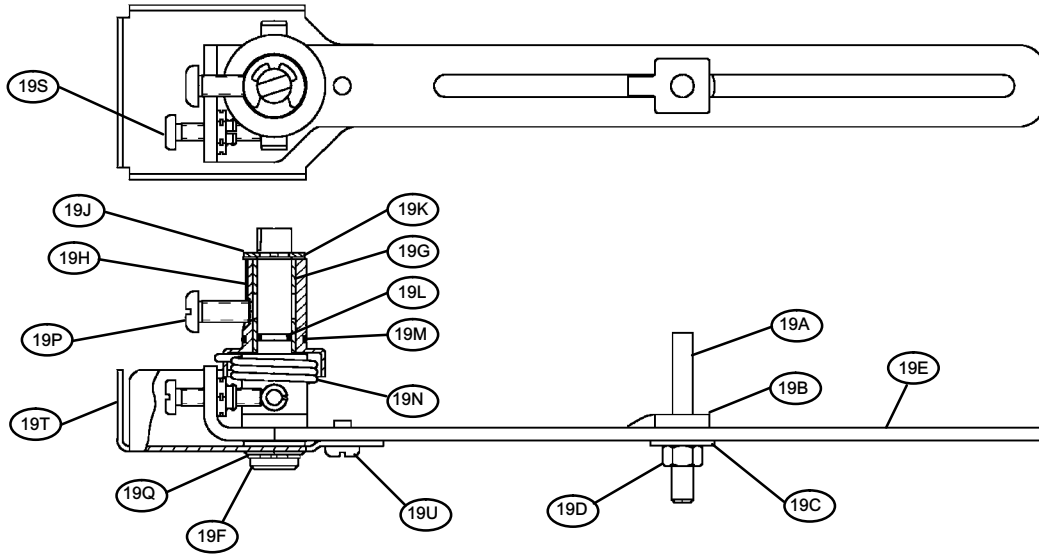
Рис. 28. Узел рычага обратной связи
