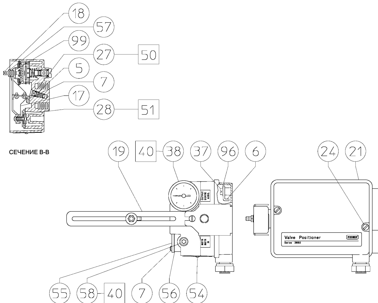
Рис. 27. Позиционер Fisher 3661 в сборе (продолжение)
