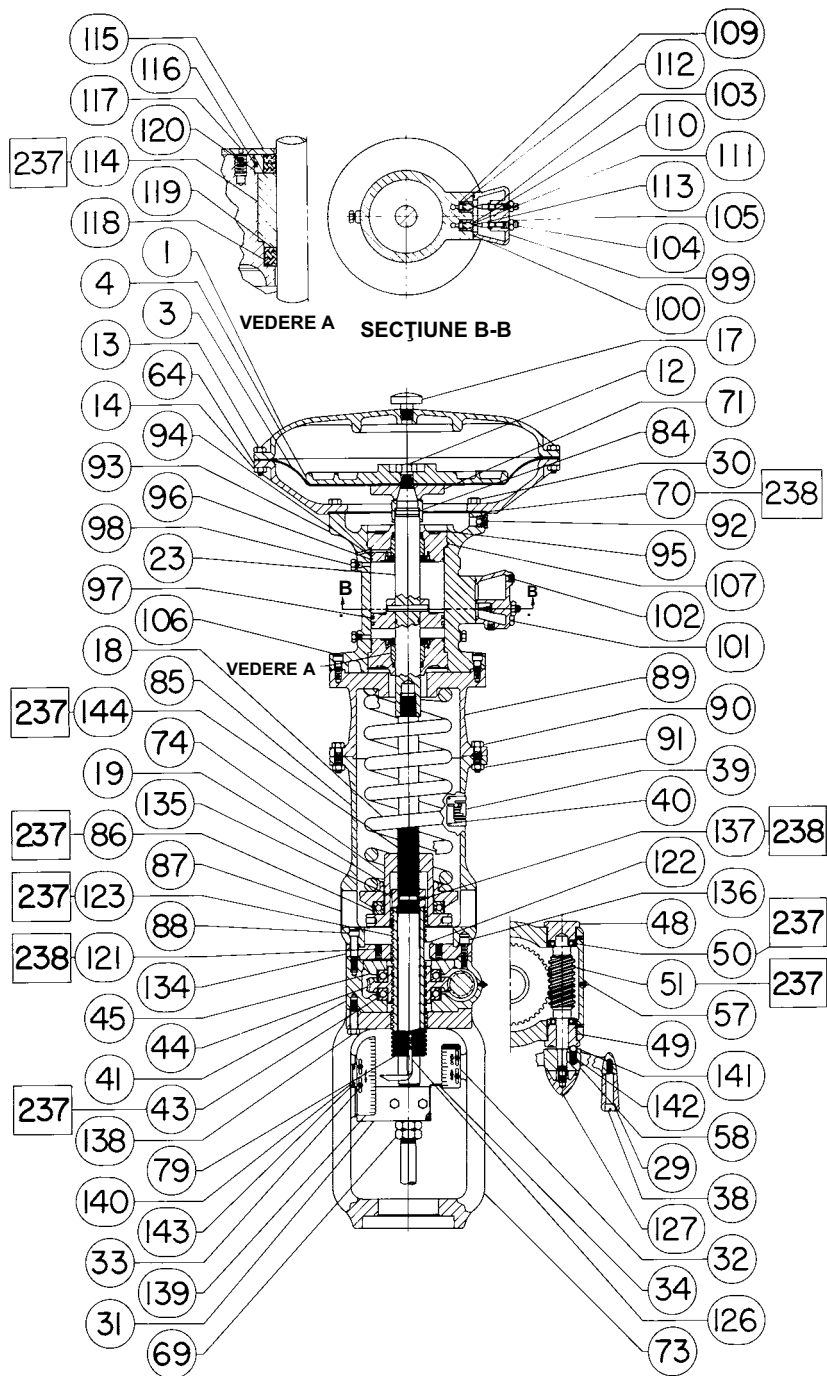
Figura 8. Actuator Fisher 667 dimensiune 80 cu roată de mână în lateral și element hidraulic de acțiune
