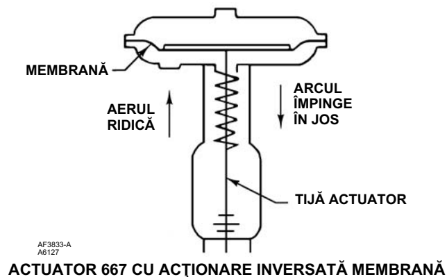
Figura 2. Reprezentare schematică Actuator Fisher 667
