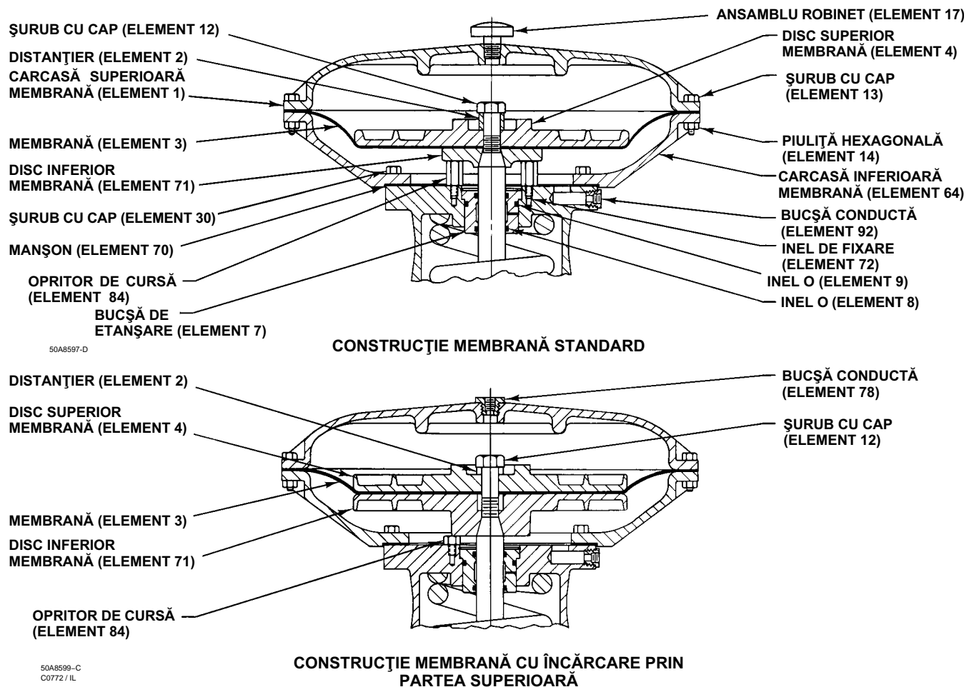
Figura 4. Construcția Actuatorului de dimensiune 80
