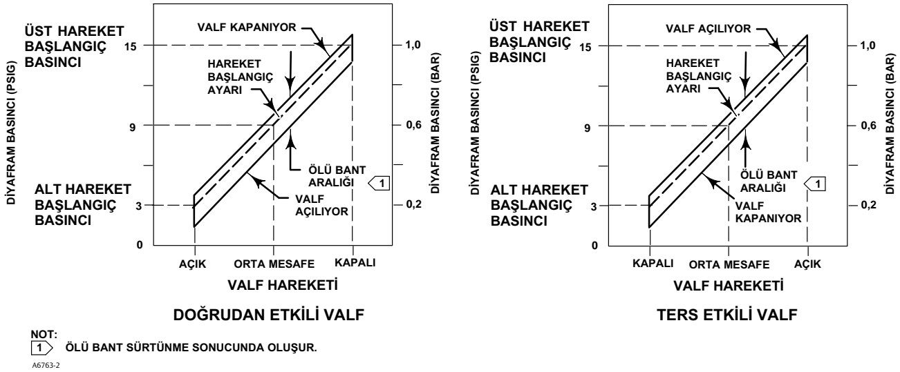
Şekil 5. Ölü Banda Tipik Valf Tepkisi
