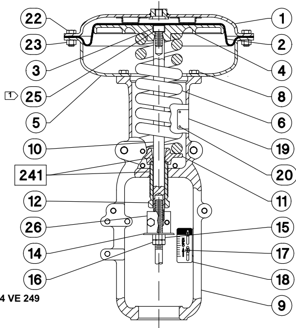
Şekil 7. 30i ila 60i Arası Ebatlı Fisher 657 Aktüatör
