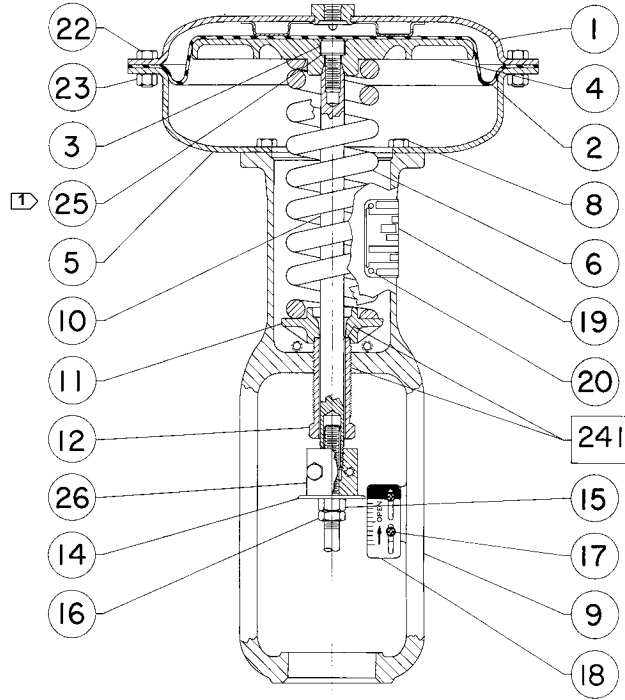
Şekil 6. 30 - 60 Arası Ebatlı Fisher 657 Aktüatörler
