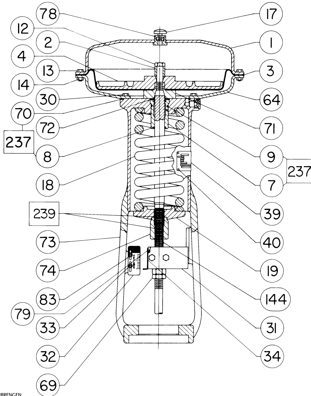
Afbeelding 10. Fisher-actuator 667, maat 87
