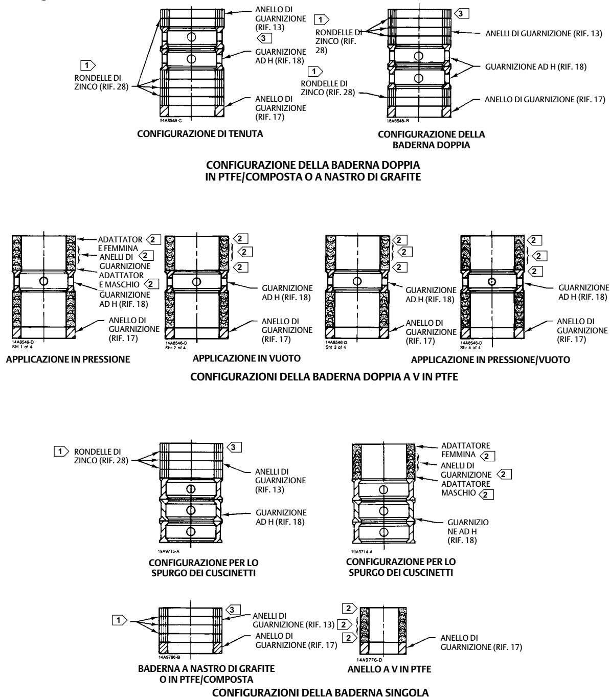
Figura 5. Configurazioni della baderna
