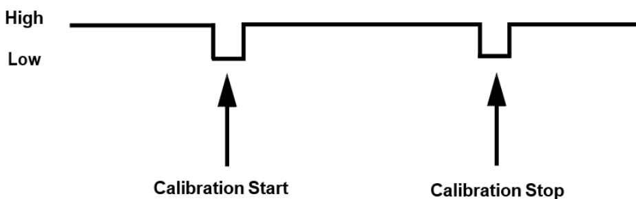
Rysunek 5-7: Bramka zbocza parametru konfiguracyjnego bramki, aktywny stan niski
