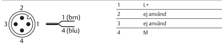
Bild 1: Anslutningsbild sensor
