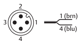
Abb. 1: Anschlussbild Sensor
