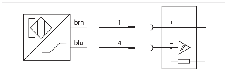
Abb. 1: Anschlussbild Sensor
