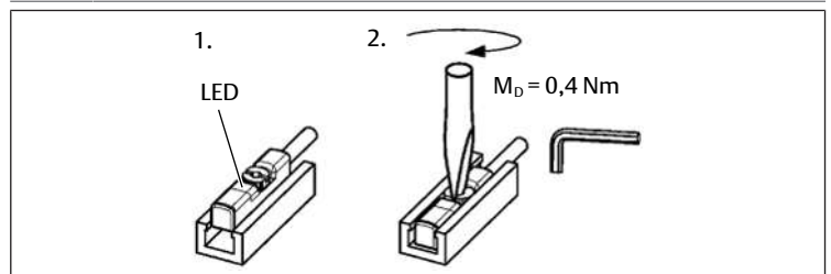
Fig. 2: Montaje del sensor
