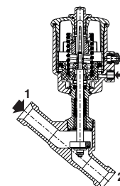
Beidseitig betätigt, Edelsthantrieb 63 mm
