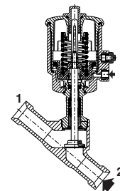
Funktion NO, Anströmung von unten, Edelsthantrieb 63 mm
