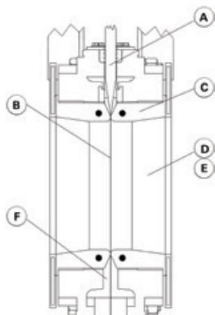
РИСУНОК 3 - ОТКРЫТОЕ ПОЛОЖЕНИЕ
