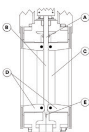
РИСУНОК 4 - ЗАКРЫТОЕ ПОЛОЖЕНИЕ
