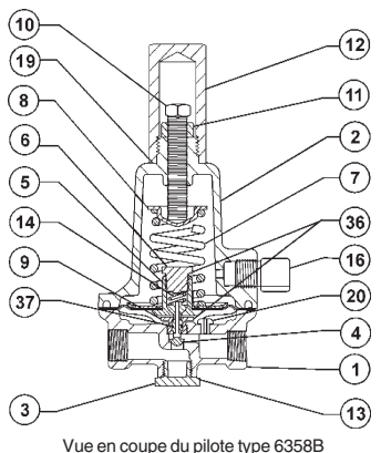
Figure 2. Pilotes types 6358 et 6358B
