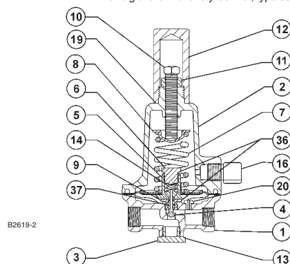
Innvendig oversikt over styreenhet, type 6358B
