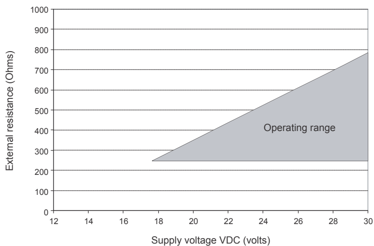
Figure C-5: Exigences de tension d'alimentation et de résistance
