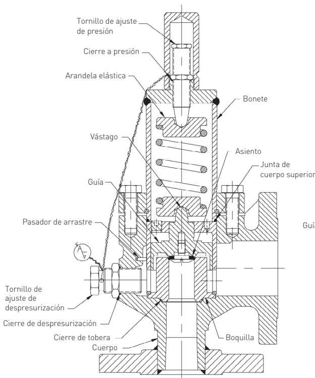
FIGURA 2 Serie 81 (Orificios F, G, H y J)
