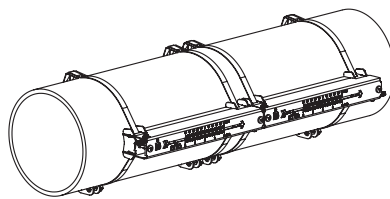
Fig. 6.15: Porta-transductor Variofix L (configuración en modo de reflexión)
