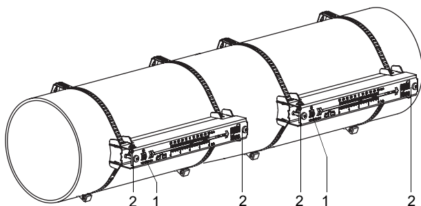
Fig. 6.37: Variofix L con transductor en la tubería
