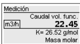
Fig. 9.2: Visualización de los valores de medición
