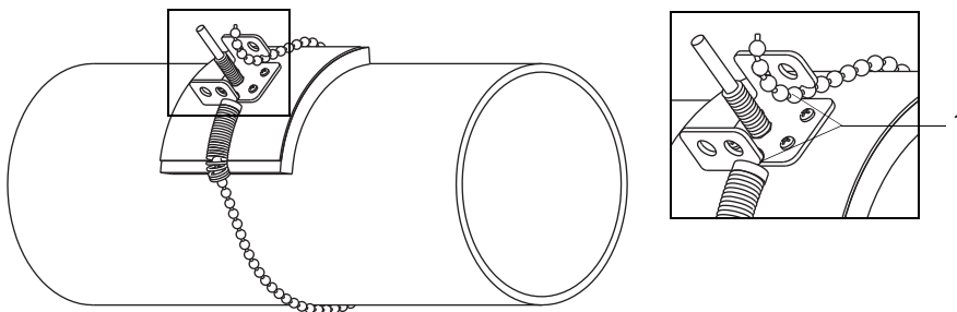
Fig. 6.68: Sensor de temperatura en la tubería
