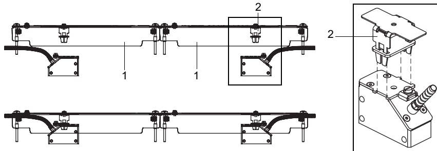
Fig. 6.34: Montaje de los transductores en las cubiertas
