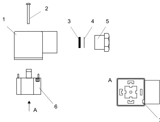
Fig. 7.20: Conector desmontado
