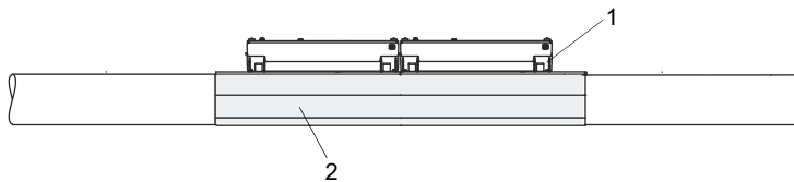
Fig. 6.5: Esteras de amortiguamiento montadas en configuración en modo de reflexión
