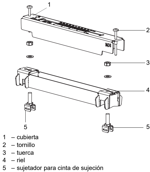
Fig. 6.16: Desmontaje del Variofix L
