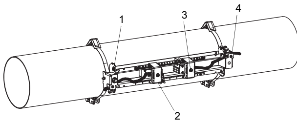
Fig. 6.60: Transductores en el riel
