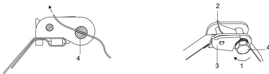
Fig. 6.32: Cierre de trinquete con cinta de sujeción
