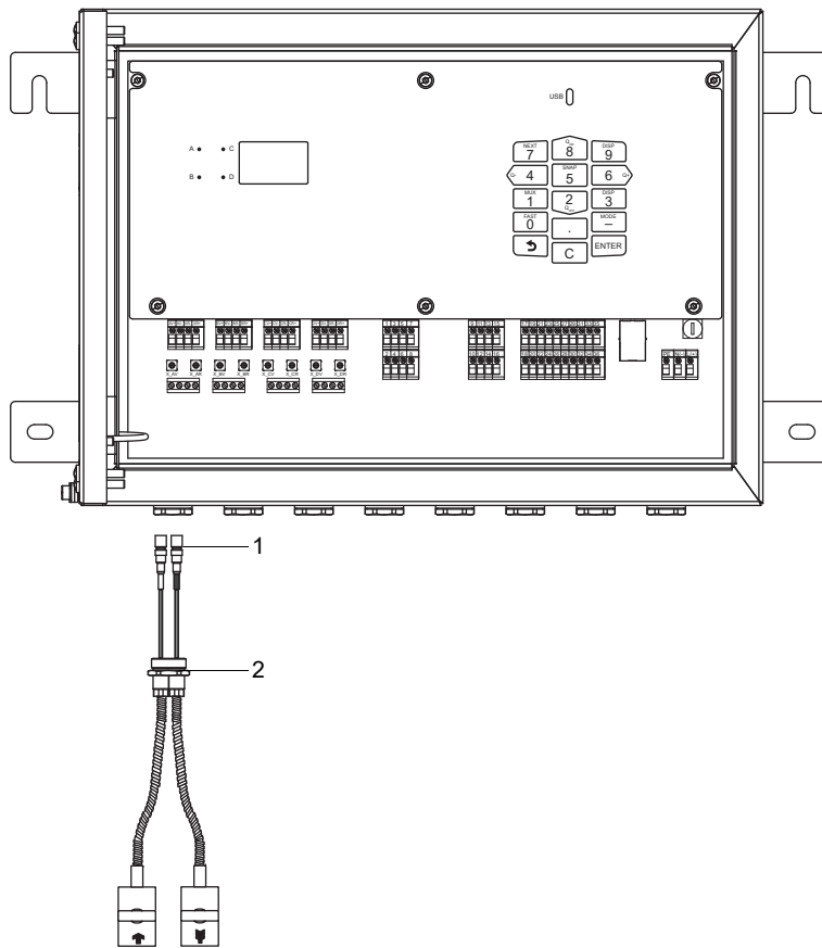
Fig. 7.2: Conexión del cable del transductor con conectores SMB al transmisor
