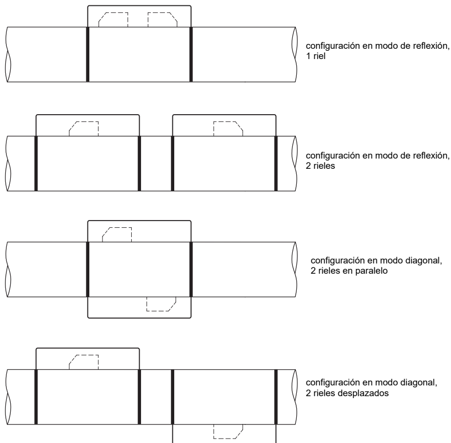
Fig. 6.12: Configuración de los transductores en rieles de montaje
