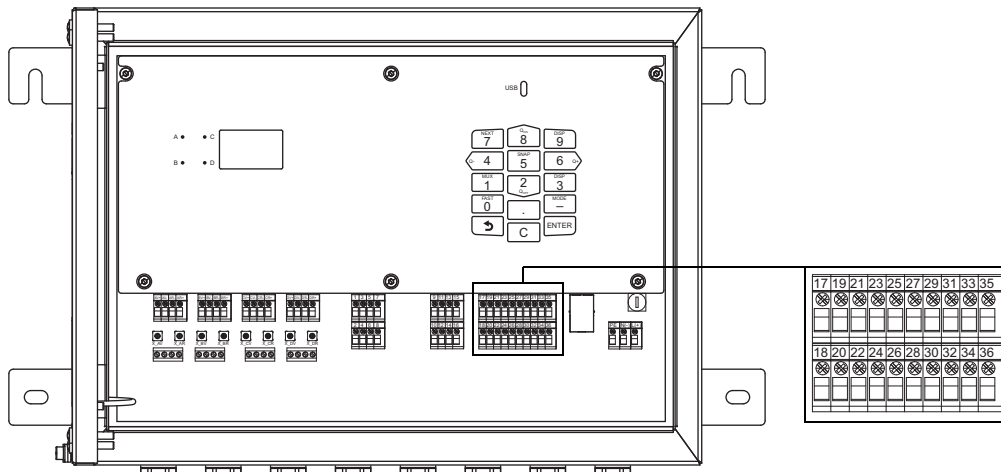
Fig. 7.14: Conexión de salidas al transmisor
