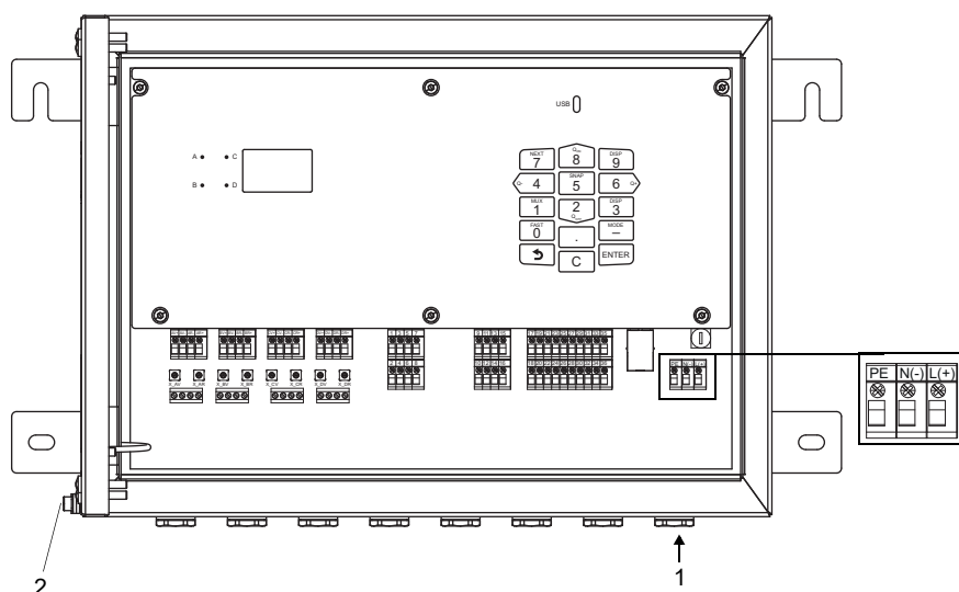
Fig. 7.12: Conexión de la fuente de alimentación al transmisor
