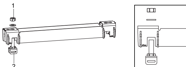
Fig. 6.26: Riel con sujetador para cinta de sujeción
