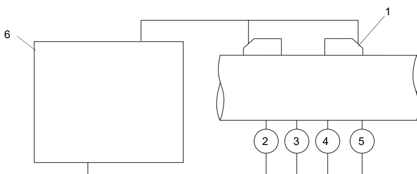
Fig. 20.1: Determinación del caudal de energía de gas durante la medición del caudal
