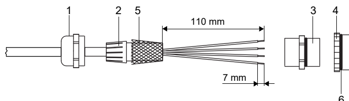
Fig. 7.18: Confección de la extensión
