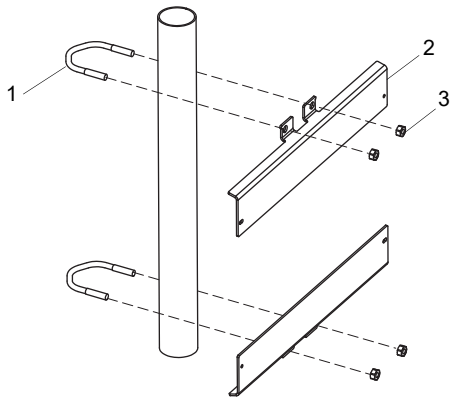
Fig. 6.3: Montaje de la chapa de soporte del instrumento
