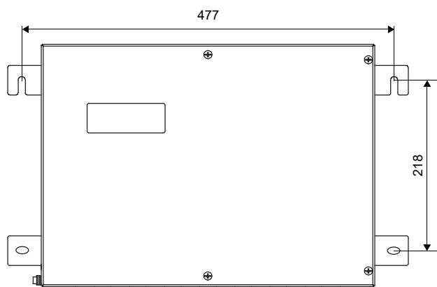
Fig. 6.2: Transmisor (dimensiones en mm)
