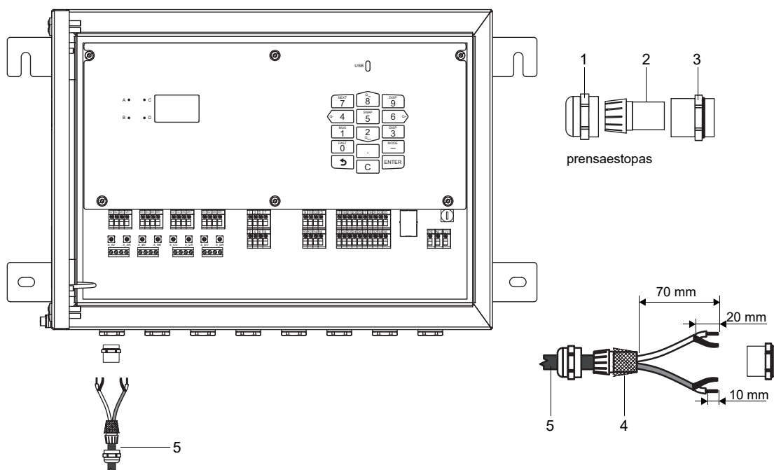
Fig. 7.5: Conexión de la extensión en el transmisor
