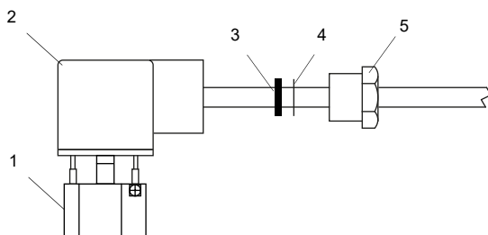
Fig. 7.24: Montaje del conector y del cable
