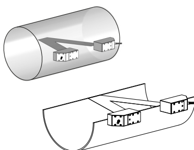
Fig. 3.7: 2 trayectorias de sonido en un plano
