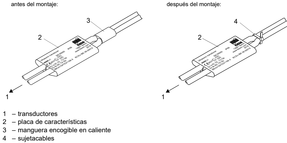
Fig. 6.13: Placa de características en el cable del transductor
