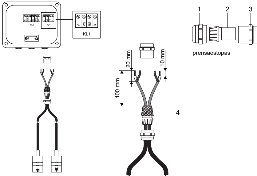
Fig. 7.7: Conexión del cable del transductor con cubierta exterior de plástico y extremos pelados
