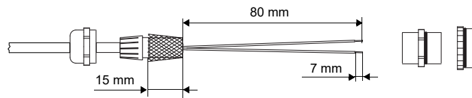
Fig. 7.29: Cable confeccionado
