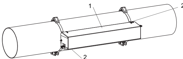
Fig. 6.61: Variofix C con transductores en la tubería
