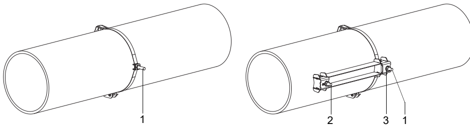
Fig. 6.27: Riel montado en un lado de la tubería
