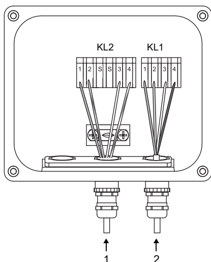
Fig. 7.19: Caja de bornes
