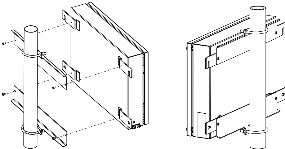
Fig. 6.4: Montaje del transmisor
