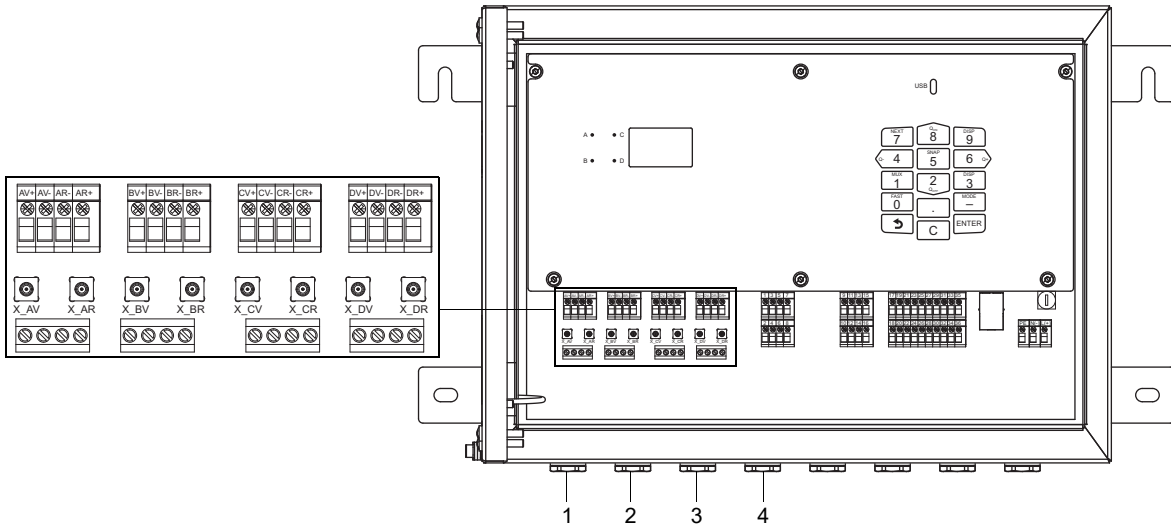
Fig. 7.1: Conexión de los transductores en el transmisor
