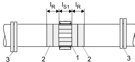
Fig. 6.10: Diámetro exterior de la tubería &gt; 900 mm
