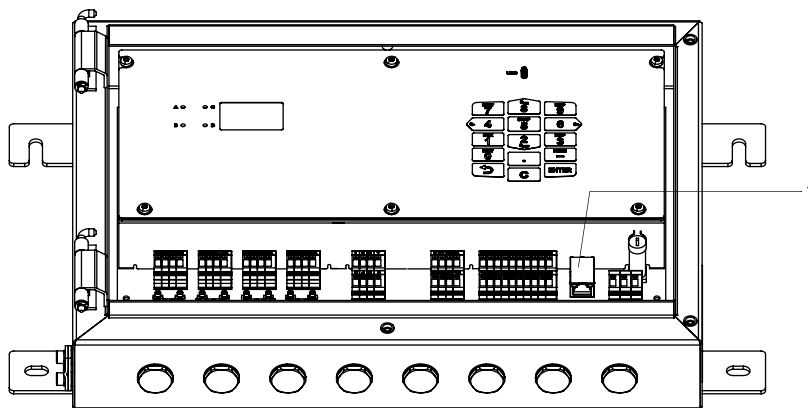
Fig. 7.31: Conexión del cable LAN
