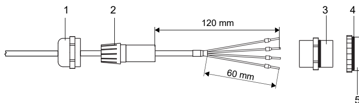
Fig. 7.17: Confección del sensor de temperatura
