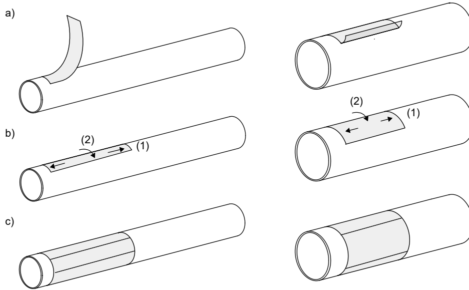
Fig. 6.8: Fijación de la esteras de amortiguamiento
