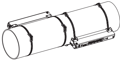
Fig. 6.14: Porta-transductor Variofix L (configuración en modo diagonal)
