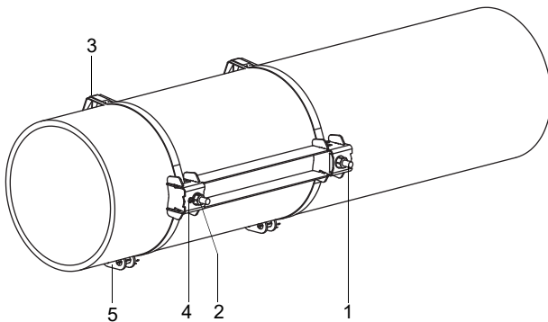
Fig. 6.28: Riel en la tubería
