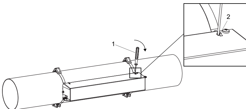
Fig. 6.62: Retiro de la cubierta
