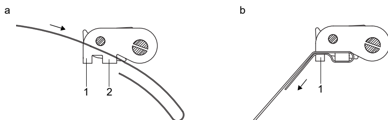
Fig. 6.44: Cierre de trinquete con cinta de sujeción
