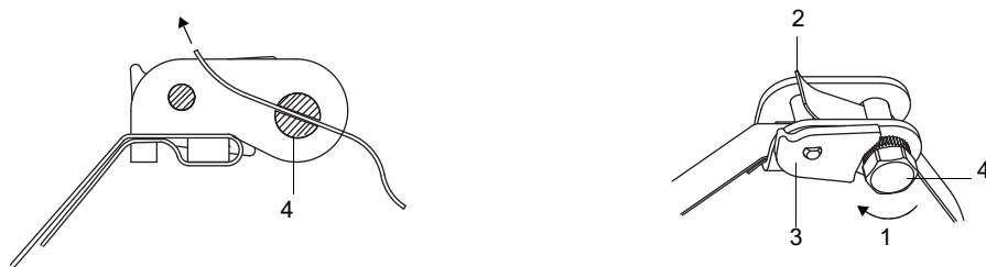
Fig. 6.57: Cierre de trinquete con cinta de sujeción
