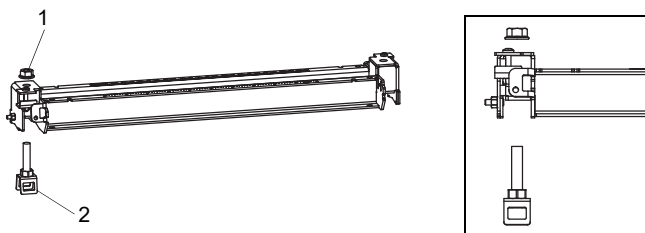
Fig. 6.51: Riel con sujetador para cinta de sujeción
