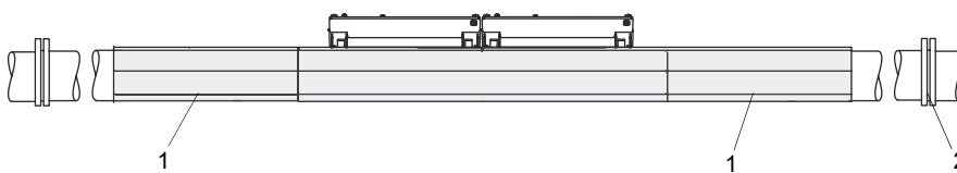
Fig. 6.6: Esteras de amortiguamiento para el transductor y la tubería en configuración en modo de reflexión
