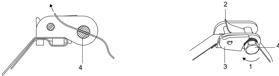
Fig. 6.50: Cierre de trinquete con cinta de sujeción
