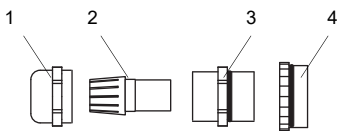
Fig. 7.28: Prensaestopas
