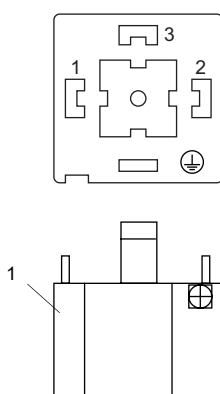
Fig. 7.23: Conexión de bornes (conector)
