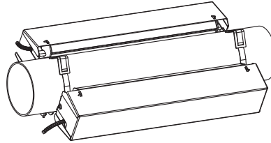
Fig. 6.39: Porta-transductores Variofix C (configuración en modo diagonal)
