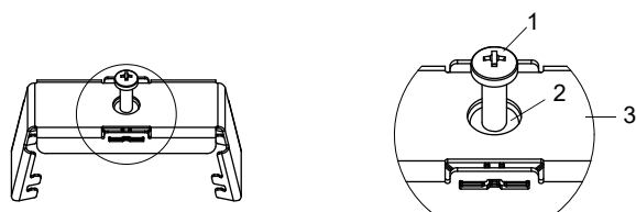
Fig. 6.59 : Étrier à ressort
