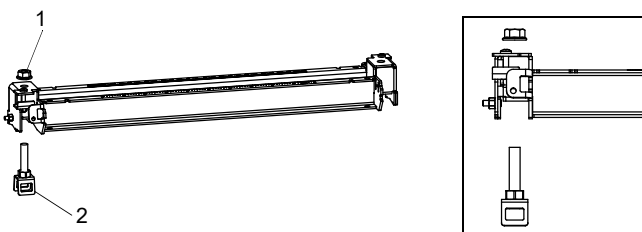
Fig. 6.51 : Rail avec pince pour bande de serrage
