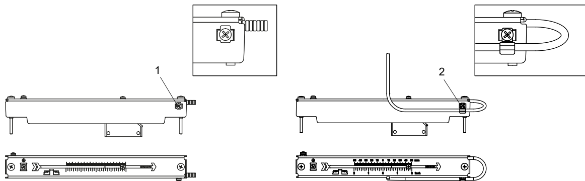
Fig. 6.36 : Fixation des câbles de capteurs
