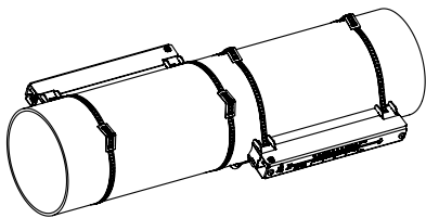
Fig. 6.14 : Fixation pour capteur Variofix L (montage diagonal)
