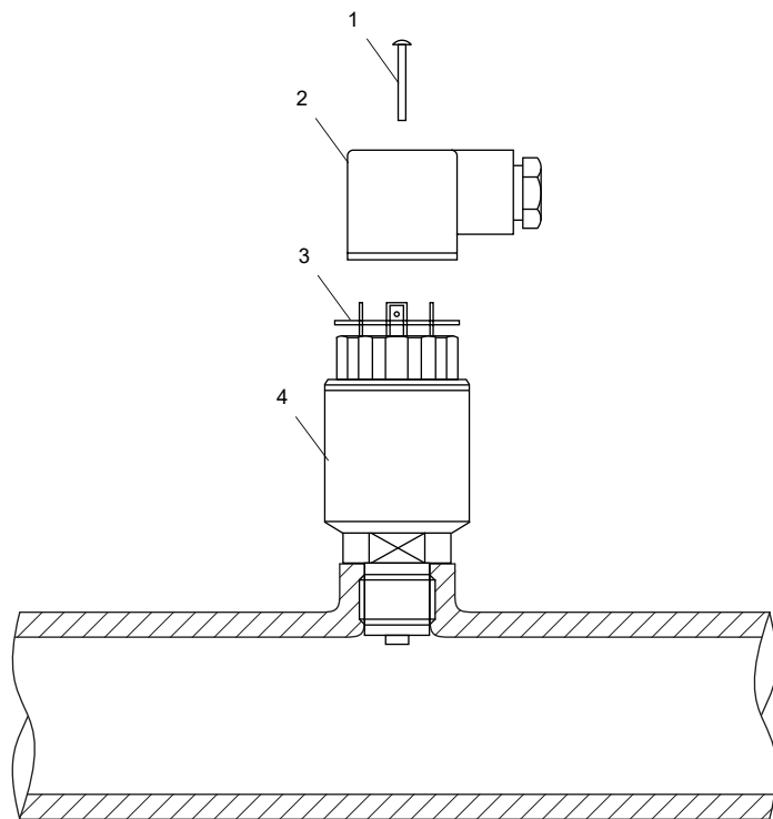
Fig. 7.25 : Fixation du connecteur
