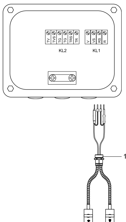
Fig. 7.8 : Raccordement du câble de capteurs avec gaine en acier inoxydable et extrémités dénudées
