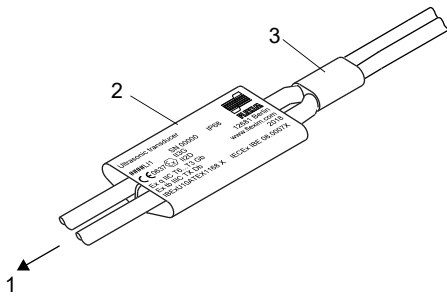
Fig. 6.13 : Plaquette signalétique au câble de capteurs
