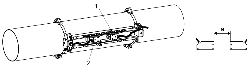
Fig. 6.58 : Capteurs dans le rail (étriers à ressort non représentés)
