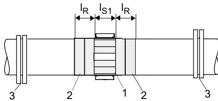
Fig. 6.10 : Diamètre extérieur de la conduite > 900 mm
