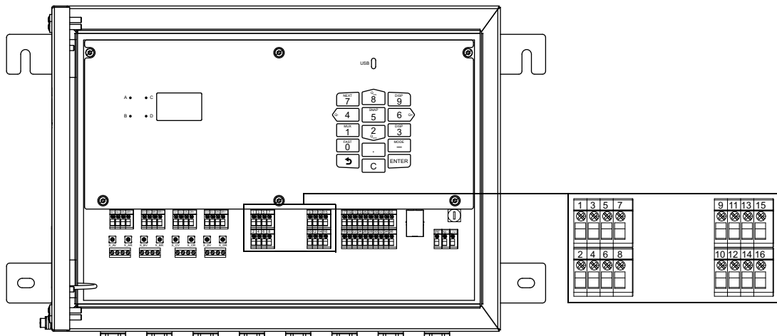
Fig. 7.27 : Raccordement des entrées au transmetteur
