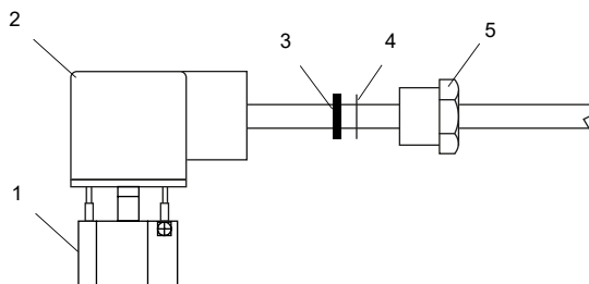
Fig. 7.24 : Montage du connecteur et du câble
