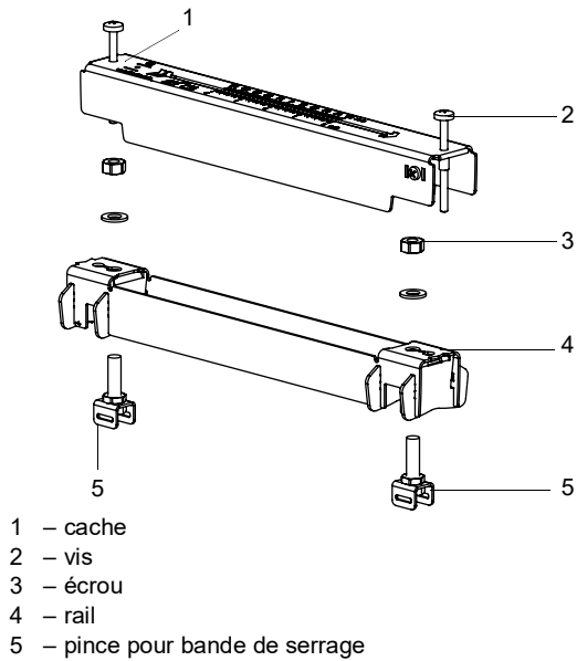
Fig. 6.16 : Démontage de la fixation Variofix L
