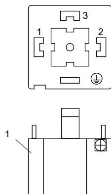
Fig. 7.23 : Brochage (connecteur)
