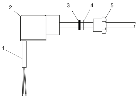
Fig. 7.21 : Montage du câble
