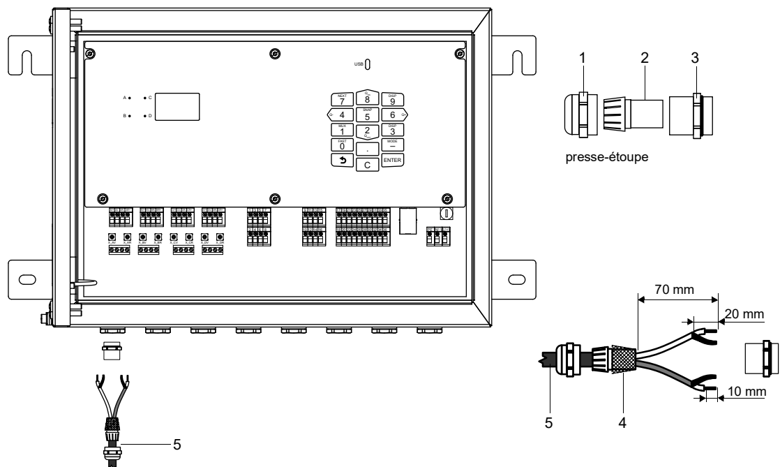
Fig. 7.5 : Raccordement de la rallonge au transmetteur
