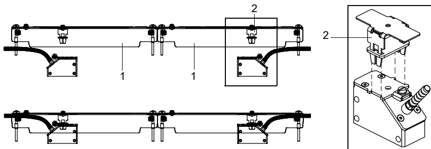
Fig. 6.34 : Montage des capteurs dans les caches
