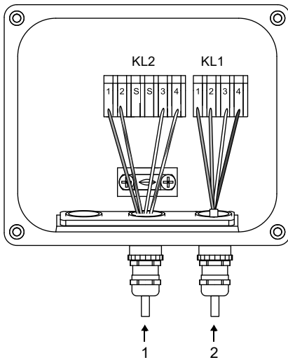
Fig. 7.19 : Boîtier de jonction
