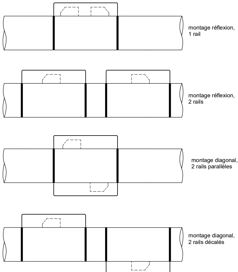
Fig. 6.12 : Disposition des capteurs dans les rails de montage
