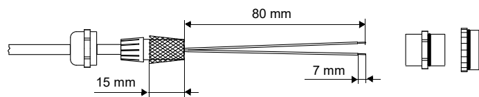
Fig. 7.29 : Câble préparé
