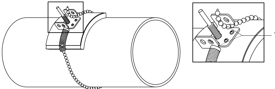
Fig. 6.68 : Sonde de température sur la conduite
