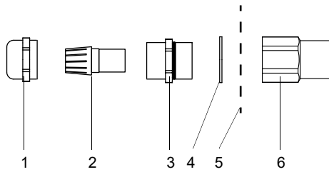
Fig. 7.32 : Presse-étoupe
