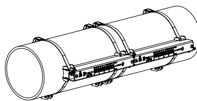
Fig. 6.15 : Fixation pour capteur Variofix L (montage réflexion)
