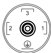
Fig. 7.26 : Broches de contact sur le transmetteur de pression
