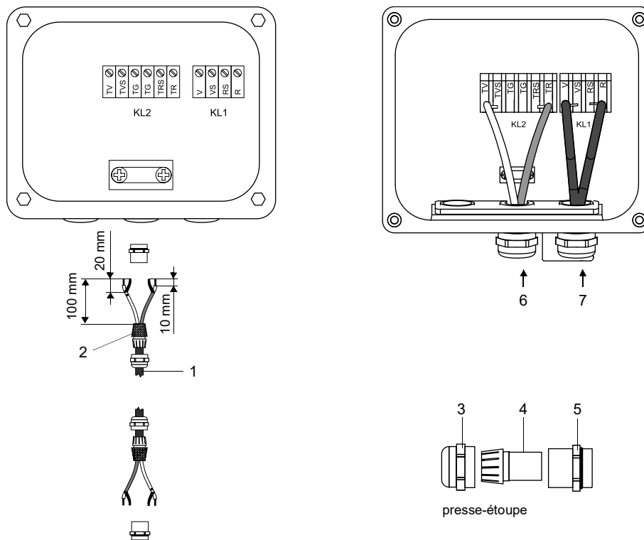
Fig. 8.9 : Raccordement de la rallonge au boîtier de jonction (sans séparation de potentiel)
