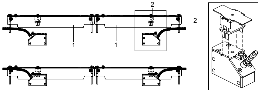
Fig. 7.31 : Montage des capteurs dans les caches
