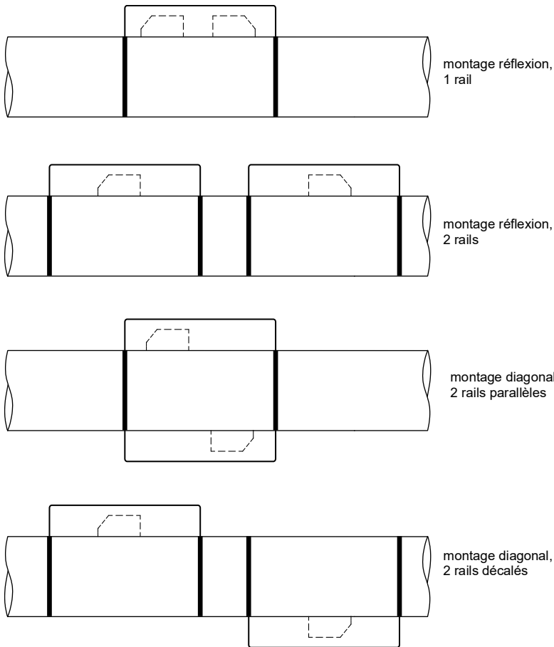
Fig. 7.9 : Disposition des capteurs dans les rails de montage
