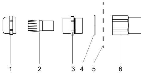
Fig. 8.25 : Presse-étoupe
