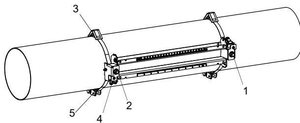
Fig. 7.50 : Rail sur la conduite
