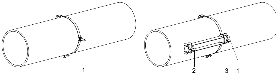
Fig. 7.24 : Rail fixé d'un côté à la conduite
