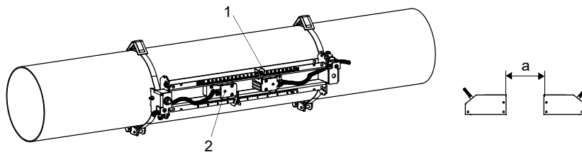
Fig. 7.55 : Capteurs dans le rail (étriers à ressort non représentés)
