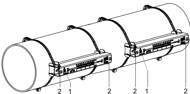
Fig. 7.34 : Variofix L avec capteurs sur la conduite
