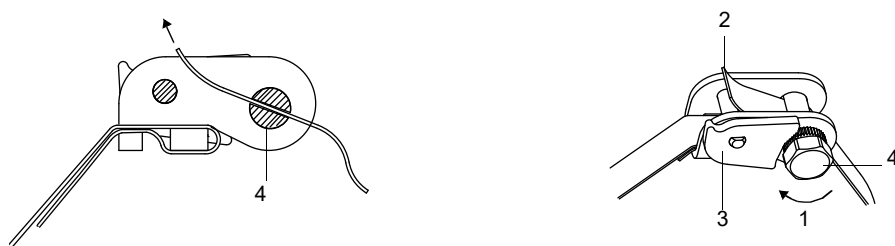
Fig. 7.29 : Fermoir à cliquet avec bande de serrage
