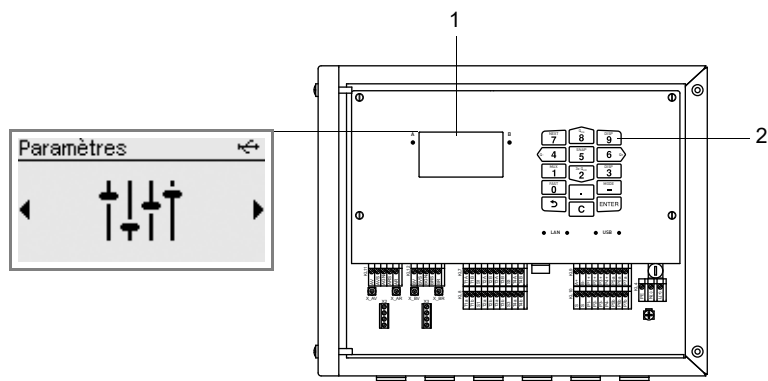
Fig. 5.2 : Panneau de commande du transmetteur
