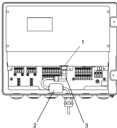
Fig. 8.26 : Raccordement du câble LAN
