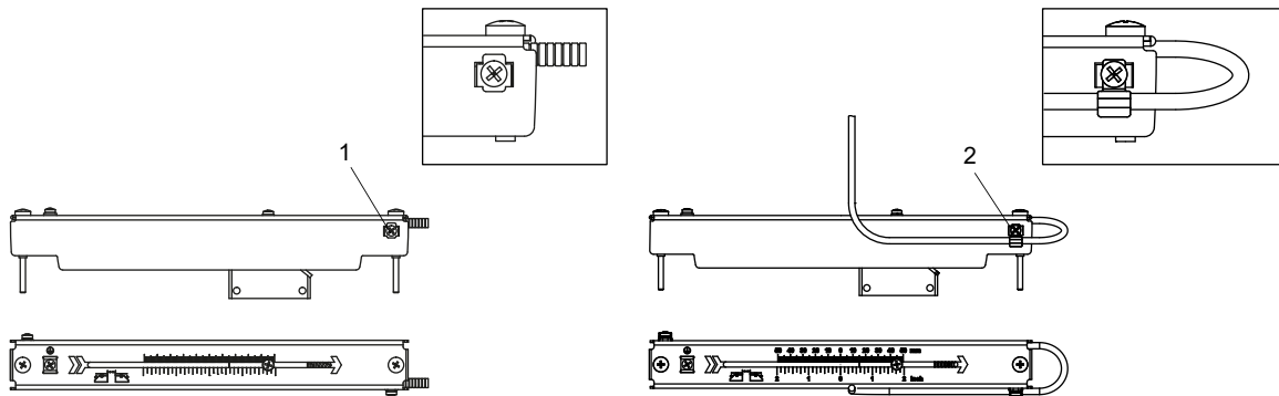
Fig. 7.33 : Fixation des câbles de capteurs
