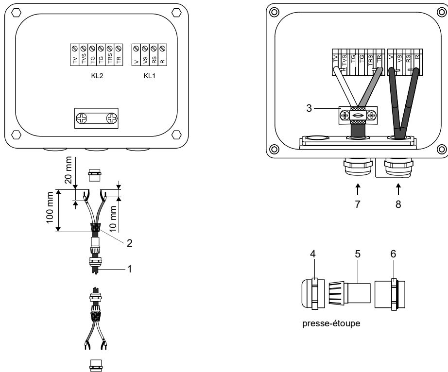
Fig. 8.10 : Raccordement de la rallonge au boîtier de jonction (avec séparation de potentiel)
