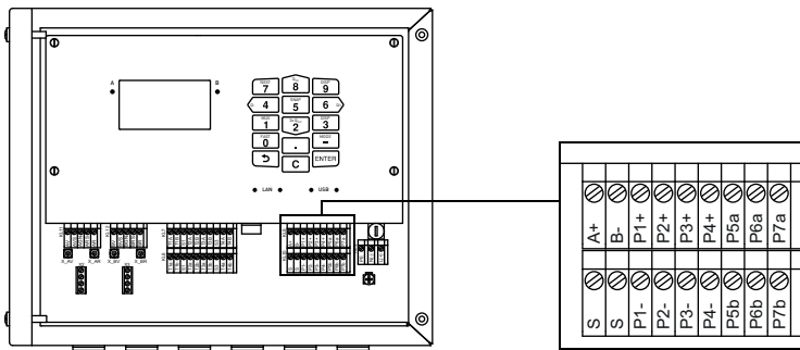
Fig. 8.16 : Raccordement des sorties au transmetteur
