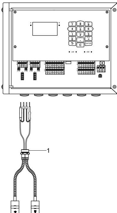
Fig. 8.4 : Raccordement du câble de capteurs avec gaine en acier inoxydable et extrémités dénudées au transmetteur
