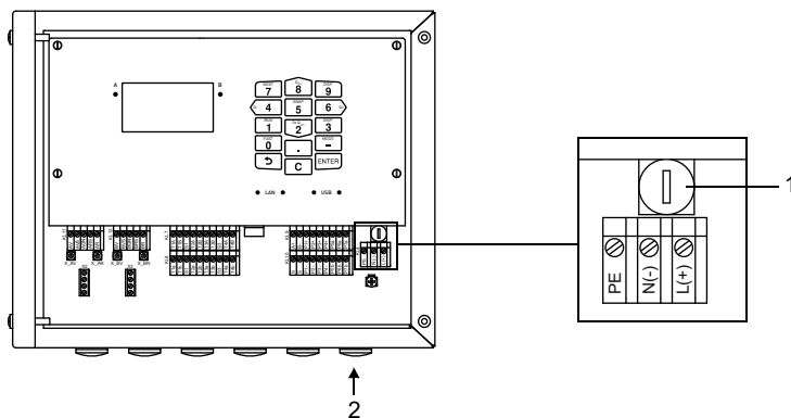
Fig. 8.13 : Raccordement de l'alimentation en tension au transmetteur
