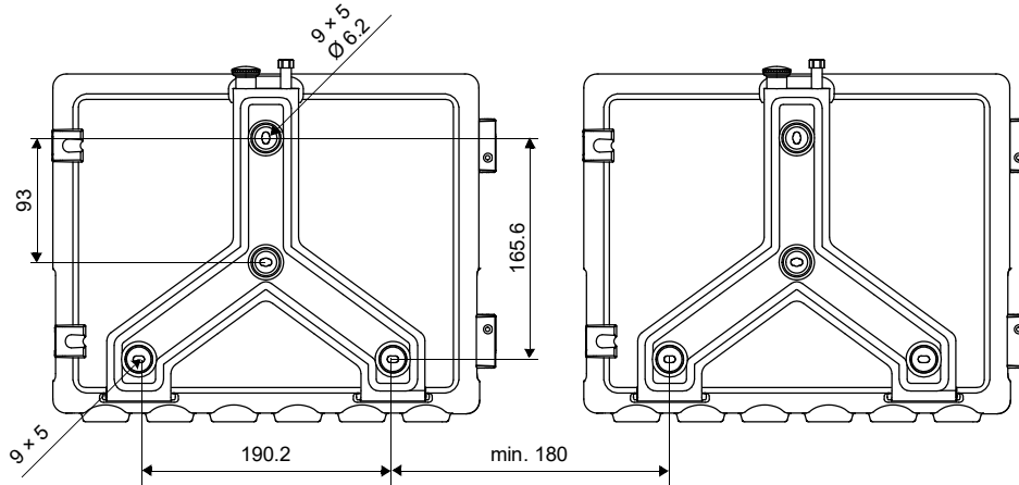
Fig. 7.4 : Transmetteur (dimensions en mm)
