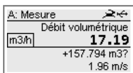
Fig. 5.4 : Témoins d'état (ligne 1)
