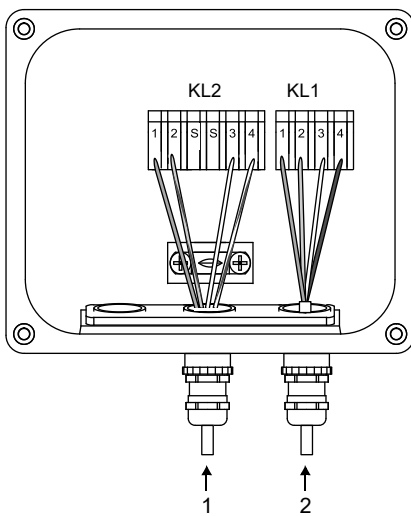
Fig. 8.22 : Boîtier de jonction
