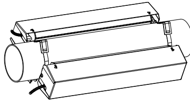
Fig. 7.36 : Fixation pour capteur Variofix C (montage diagonal)
