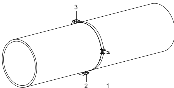
Fig. 7.17 : Bande de serrage avec pince et ressort métallique sur la conduite
