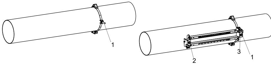
Fig. 7.49 : Rail fixé d'un côté à la conduite
