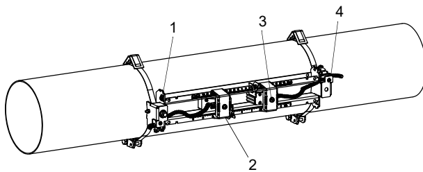
Fig. 7.57 : Capteurs dans le rail
