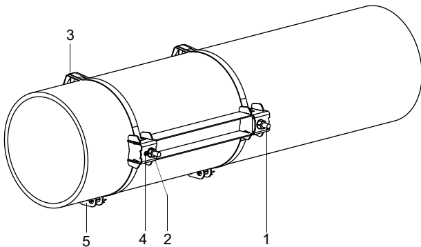
Fig. 7.25 : Rail sur la conduite
