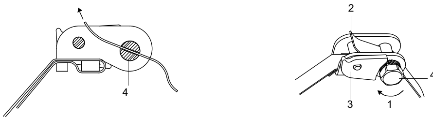
Fig. 7.54 : Fermeture à cliquet avec bande de serrage
