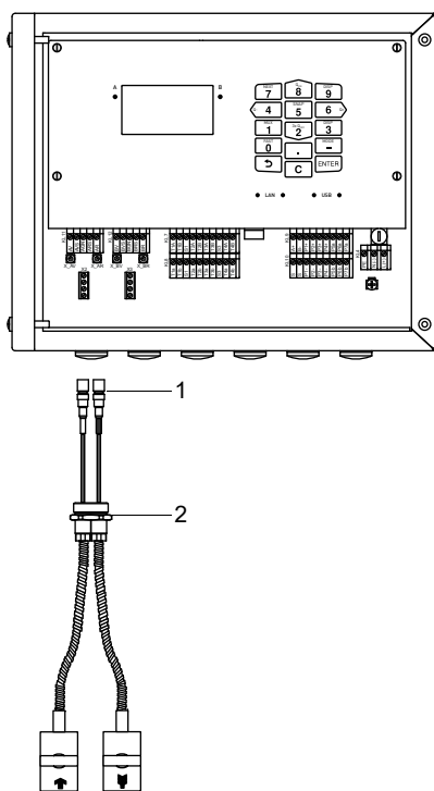
Fig. 8.2 : Raccordement du câble de capteurs avec connecteurs SMB au transmetteur
