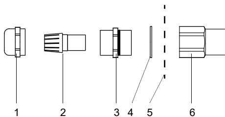
Fig. 8.14 : Presse-étoupe pour boîtier en acier inoxydable
