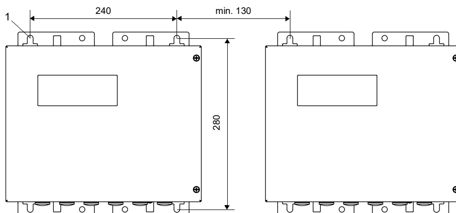
Fig. 7.3 : Transmetteur (dimensions en mm)
