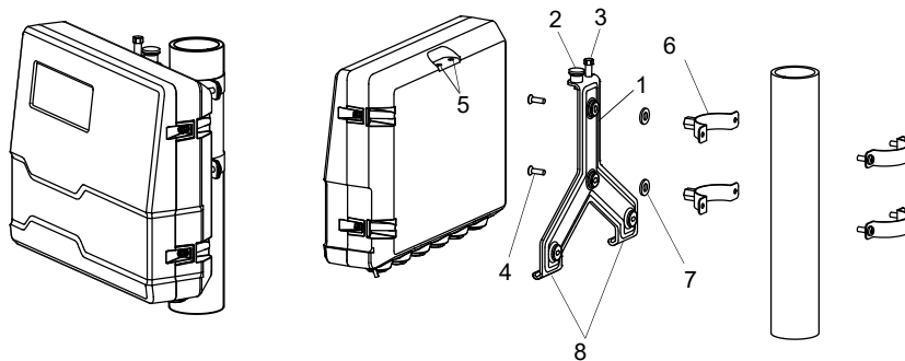
Fig. 7.7 : Vue de montage
