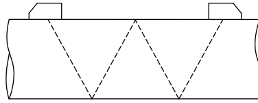
Fig. 4.5 : Montage réflexion à 1 faisceau et 4 trajets du son
