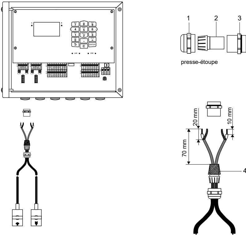
Fig. 8.3 : Raccordement du câble de capteurs avec gaine plastique et extrémités dénudées au transmetteur
