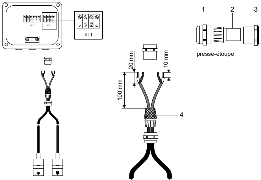
Fig. 8.7 : Raccordement du câble de capteurs avec gaine plastique et extrémités dénudées
