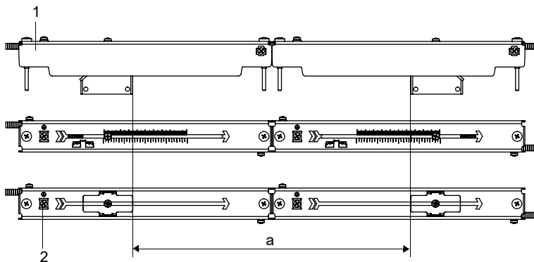
Fig. 7.32 : Réglage de l'écart entre les capteurs
