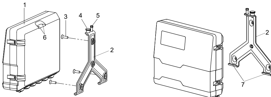
Fig. 7.5 : Vue de montage
