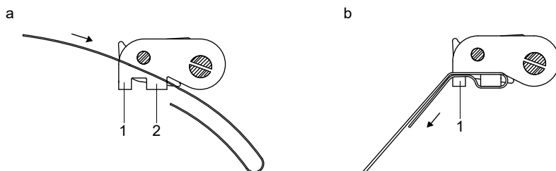
Fig. 7.41 : Fermeture à cliquet avec bande de serrage
