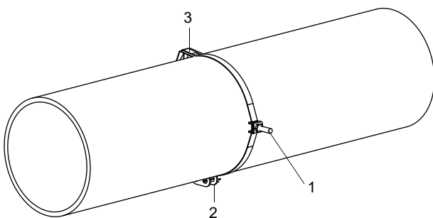
Fig. 7.42 : Bande de serrage avec pince et ressort métallique sur la conduite
