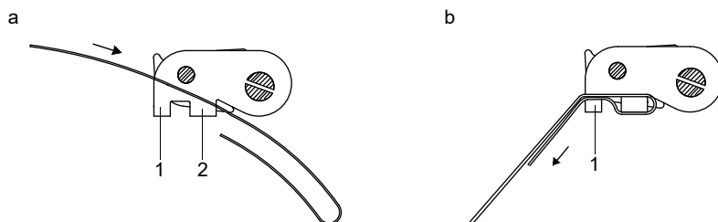
Fig. 7.16 : Fermeture à cliquet avec bande de serrage
