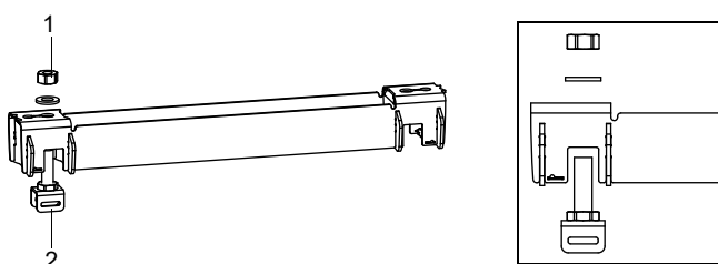
Fig. 6.20 : Rail avec pince pour bande de serrage
