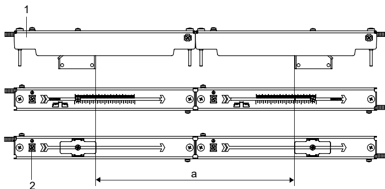
Fig. 6.29 : Réglage de l'écart entre les capteurs
