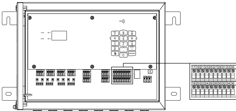
Fig. 7.14 : Raccordement des sorties au transmetteur
