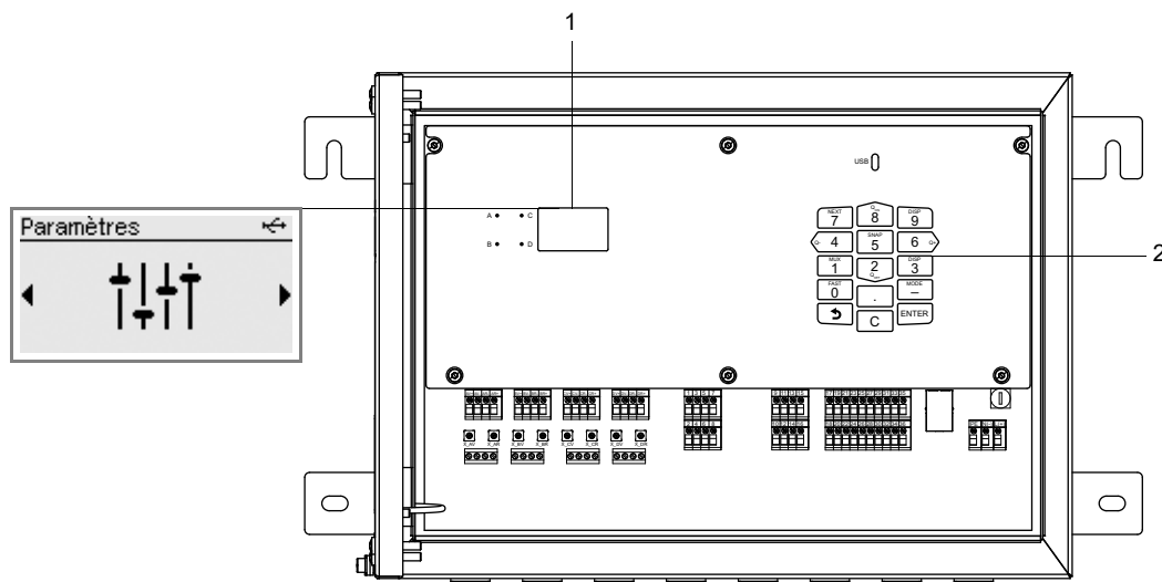
Fig. 4.2 : Panneau de commande du transmetteur
