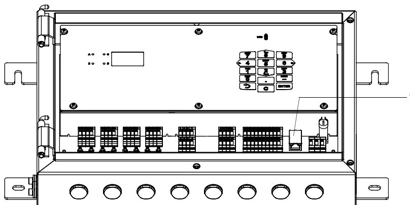
1 – interface LAN
