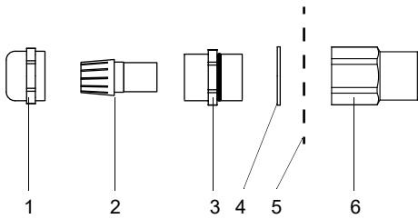
Fig. 7.22 : Presse-étoupe
