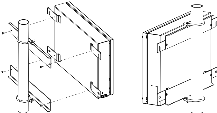
Fig. 6.4 : Montage du transmetteur
