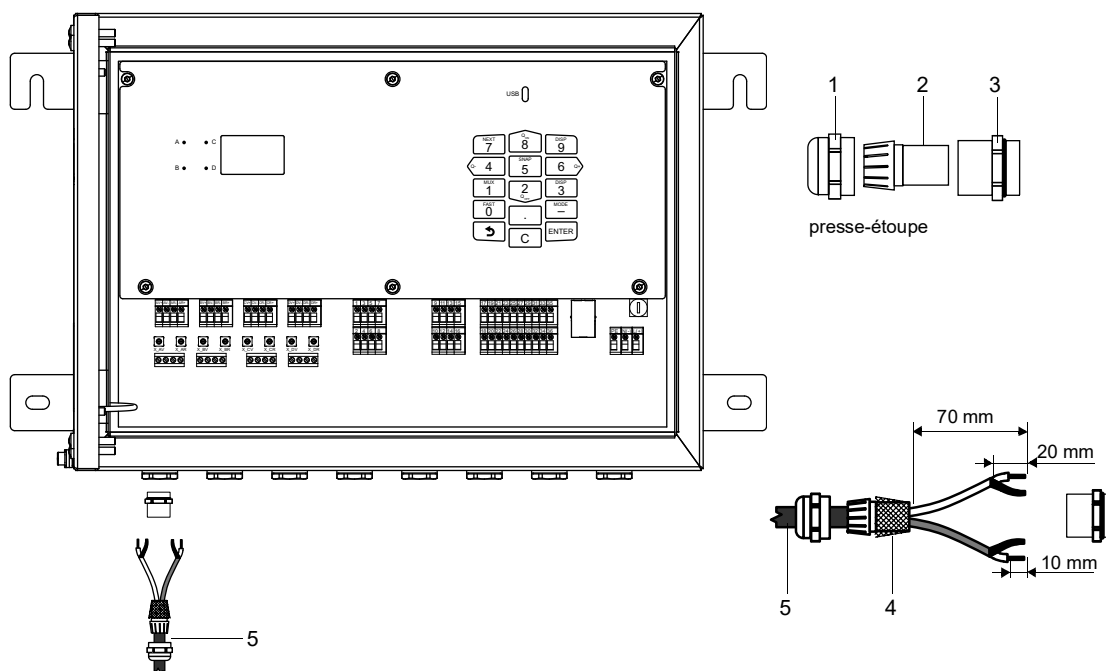
Fig. 7.5 : Raccordement de la rallonge au transmetteur
