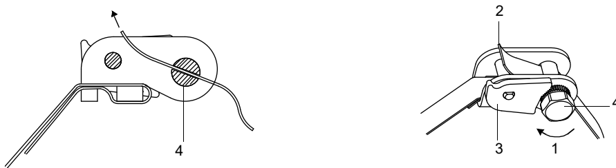
Fig. 6.44 : Fermeur à cliquet avec bande de serrage
