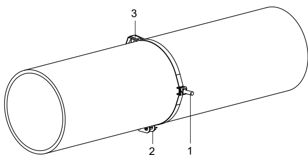
Fig. 6.14 : Bande de serrage avec pince et ressort métallique sur la conduite
