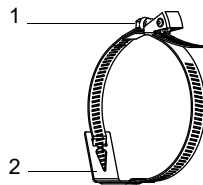
Fig. 6.16 : Bande de serrage avec fermetoir rapide et ressort métallique
