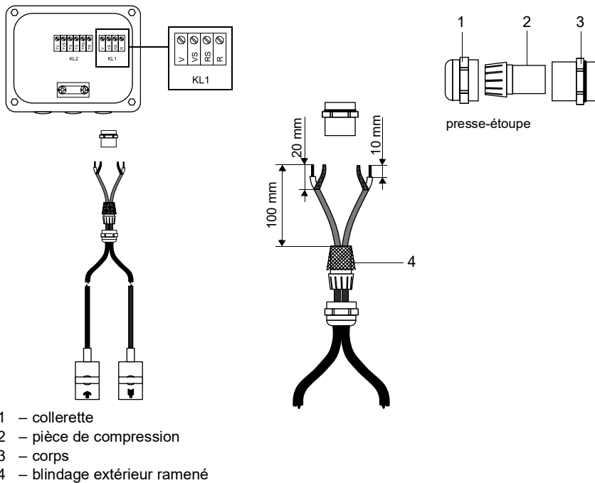
Fig. 7.7 : Raccordement du câble de capteurs avec gaine plastique et extrémités dénudées
