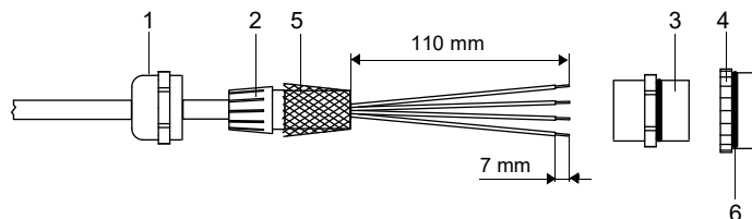
Fig. 7.18 : Préparation de la rallonge
