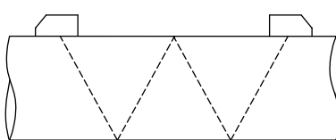
Fig. 3.6 : Montage réflexion à 1 faisceau et 4 trajets du son
