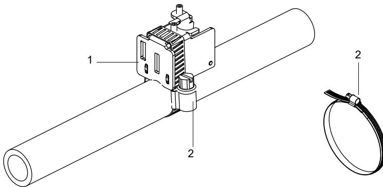
Fig. 6.57 : Capteur dans sa coquille de montage, monté à l'aide d'une bande de serrage avec fermoir
