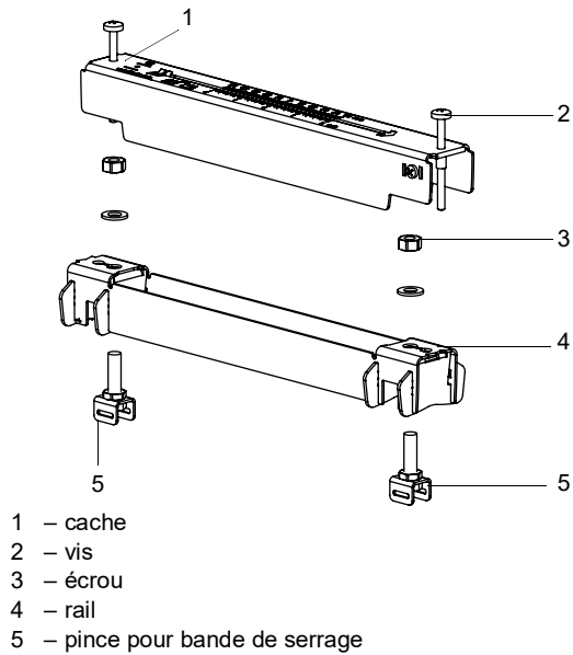
Fig. 6.10 : Démontage de la fixation Variofix L
