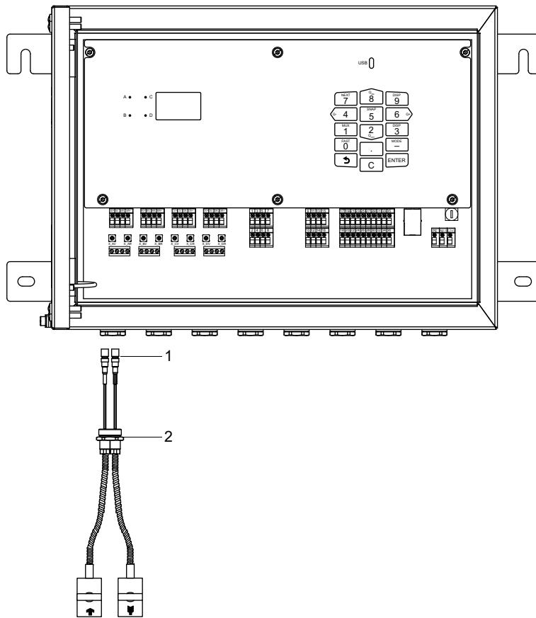
Fig. 7.2 : Raccordement du câble de capteurs avec connecteurs SMB au transmetteur
