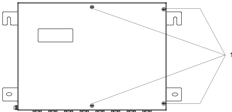
Fig. 6.1 : Transmetteur
