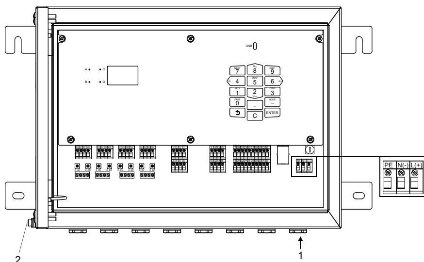
Fig. 7.12 : Raccordement de l'alimentation en tension au transmetteur
