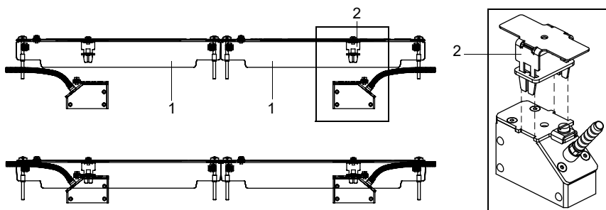
Fig. 6.28 : Montage des capteurs dans les caches
