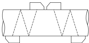
Fig. 3.5 : Montage diagonal à 2 faisceaux et 3 trajets du son
