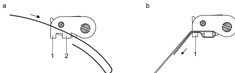
Fig. 6.38 : Fermeir à cliquet avec bande de serrage
