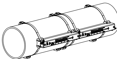
Fig. 6.9 : Fixation pour capteur Variofix L (montage réflexion)
