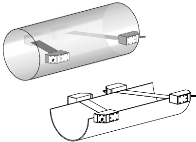
Fig. 3.7 : 2 faisceaux dans un plan
