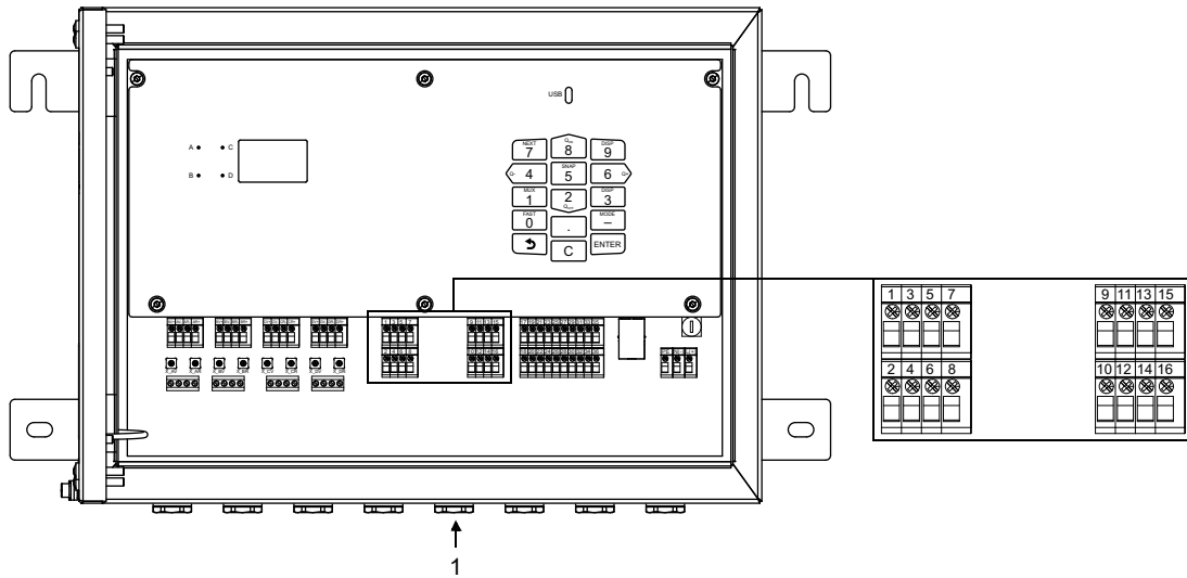
Fig. 7.16 : Raccordement des sondes de température au transmetteur
