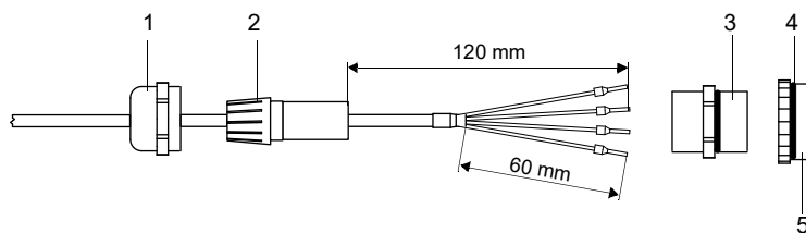
Fig. 7.17 : Préparation de la sonde de température
