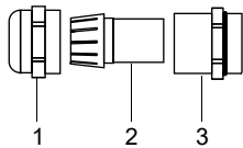
Fig. 7.13 : Presse-étoupe
