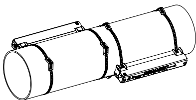
Fig. 6.8 : Fixation pour capteur Variofix L (montage diagonal)
