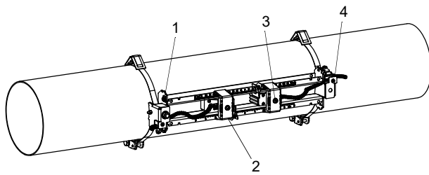
Fig. 6.54 : Capteurs dans le rail
