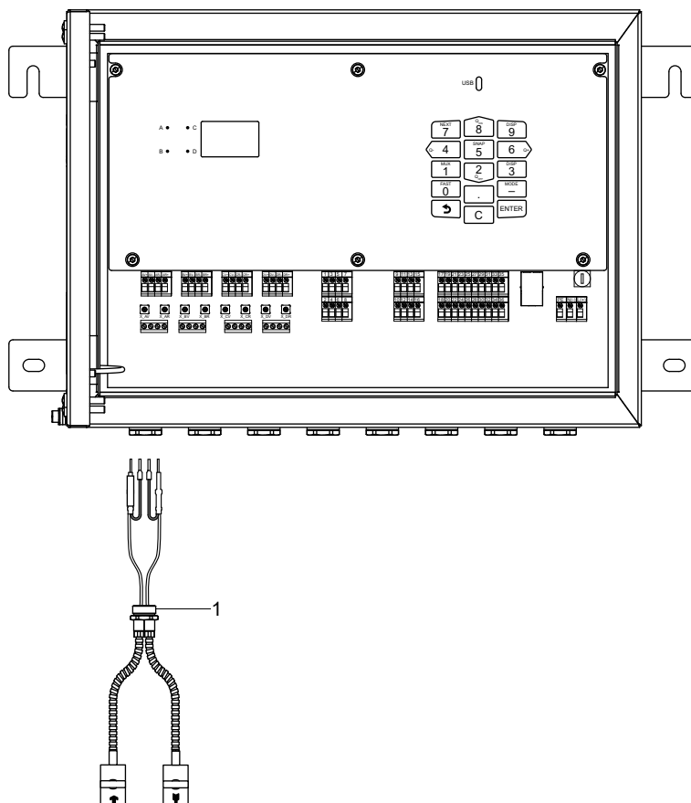
1 – presse-étoupe
