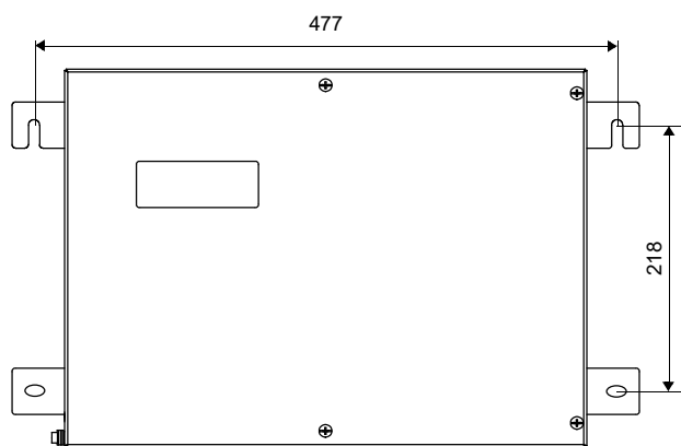
Fig. 6.2 : Transmetteur (dimensions en mm)
