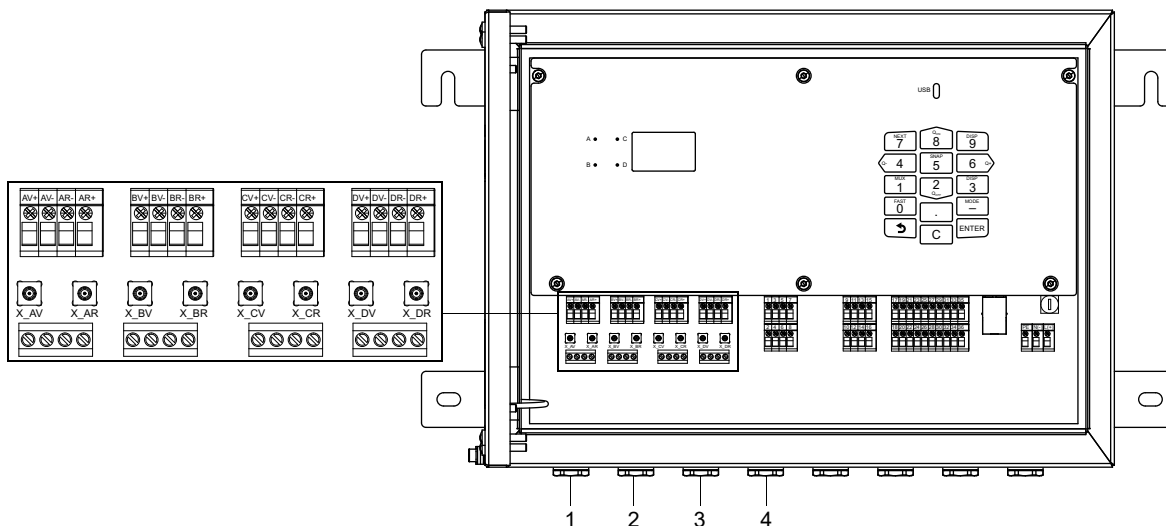
Fig. 7.1 : Raccordement des capteurs au transmetteur
