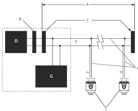
Obrázok 3-3: Typická konfigurácia pre pripojenie zbernice PROFIBUS do siete
