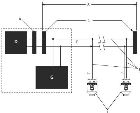
Obrázok 3-2: Typická konfigurácia pre pripojenie zbernice do siete
