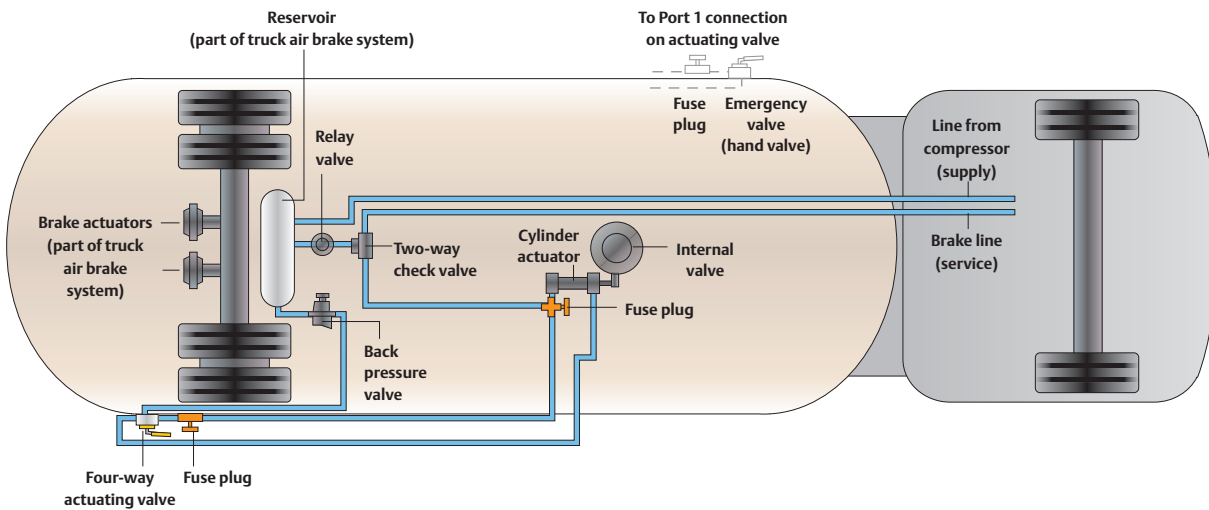
CONEXIÓN DE INTERBLOQUEO DE AIRE EN CAMIÓN CORTO
