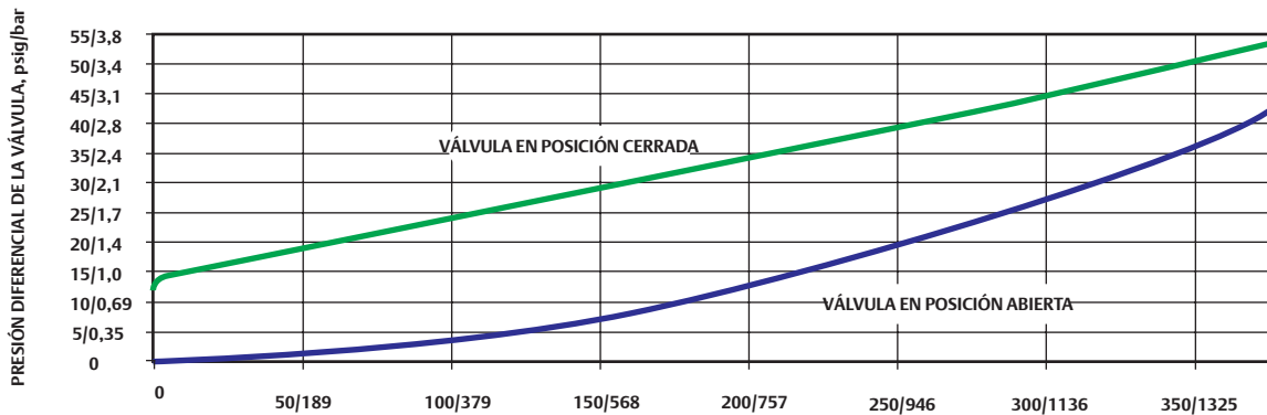
Tipo C477-16 curva típica de retorno de caudal
