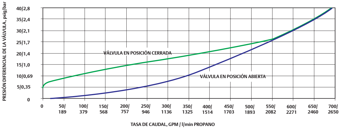
Tipo C477-24 curva típica de retorno de caudal
