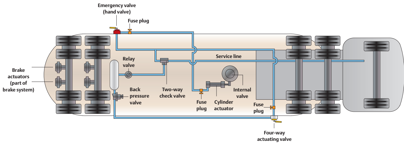
CONEXIÓN DE INTERBLOQUEO DE AIRE EN CAMIÓN DE TRANSPORTE
