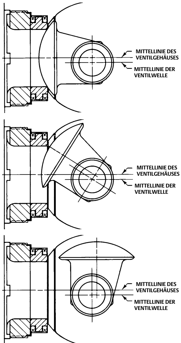
Abbildung 4. Exzentrische Drehbewegung
