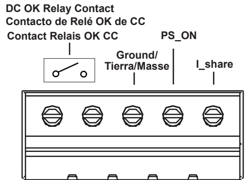
Fig. 1: Signal Connections Conexiones de Señales Connexions Signal
