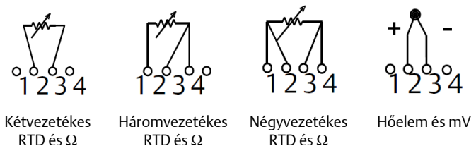
ábra 3-1: Érzékelő csatlakoztatása
