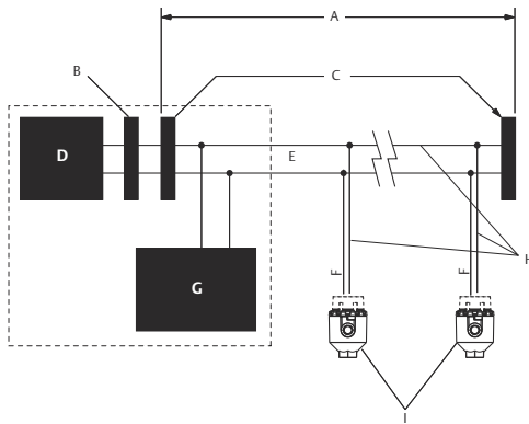
ábra 3-3: PROFIBUS hálózat tipikus elrendezése
