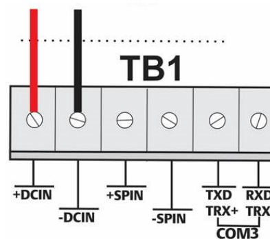
Abbildung 8. Verkabelung zur DC-Spannungsversorgung
