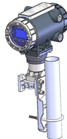
Figura 7. FB1100 con montaje en tubería
