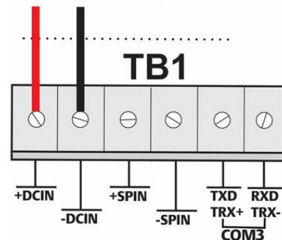
Figura 8. Cablaggio ad alimentazione c.c.
