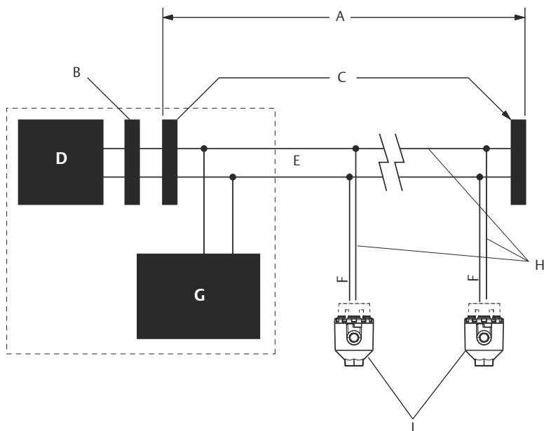
Figur 2-2. Typisk konfiguration för fältbussnätverk
